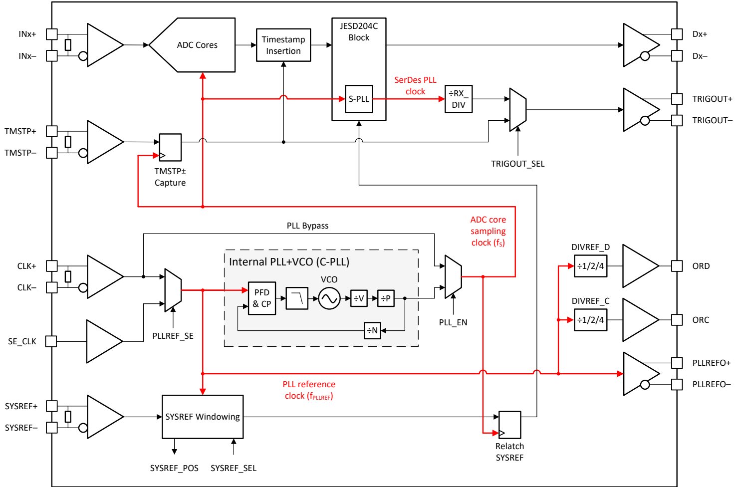
图 9-5. Clocking Subsystem
