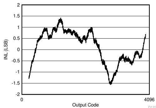
图 8-2. INL vs Code
