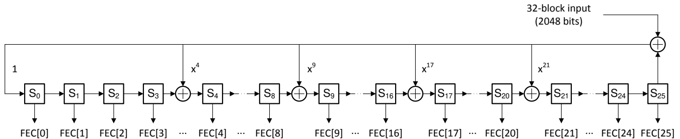
图 9-10. FEC Parity Bit Generator
