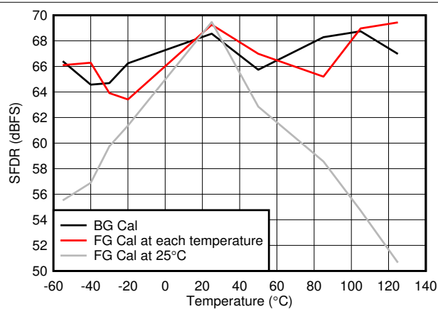
图 8-65. SFDR vs Temperature
