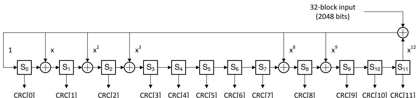
图 9-9. CRC-12 Parity Bit Generator
