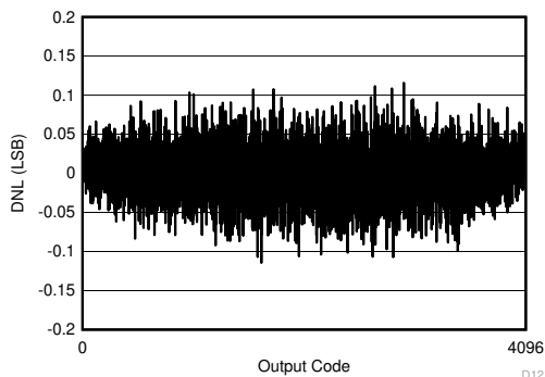
图 8-1. DNL vs Code
