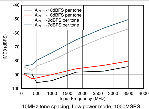
图 8-76. IMD3 vs F_{IN}
