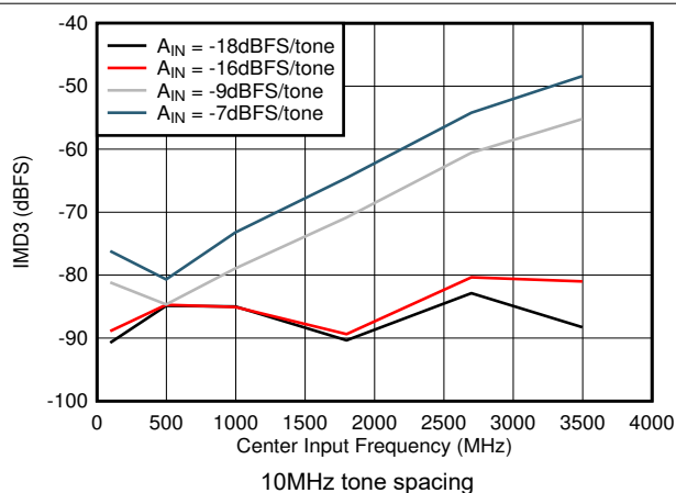
图 8-75. IMD3 vs F_{IN}
