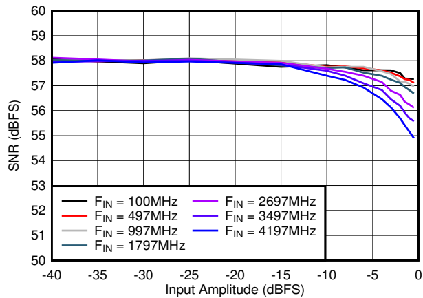
图 8-33. SNR vs A_{IN}
