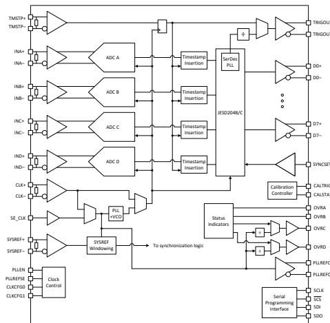
四通道器件方框图
