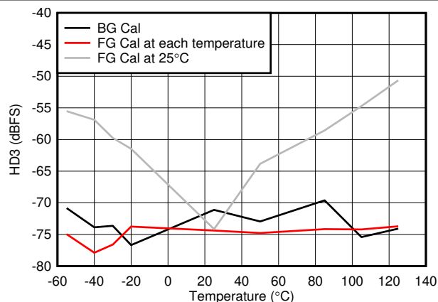
图 8-67. HD3 vs Temperature
