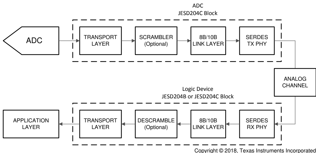
图 9-7. Simplified 8B/10B Encoded JESD204C Interface Diagram
