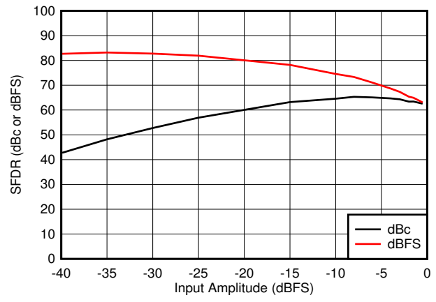
图 8-32. SFDR vs A_{IN}
