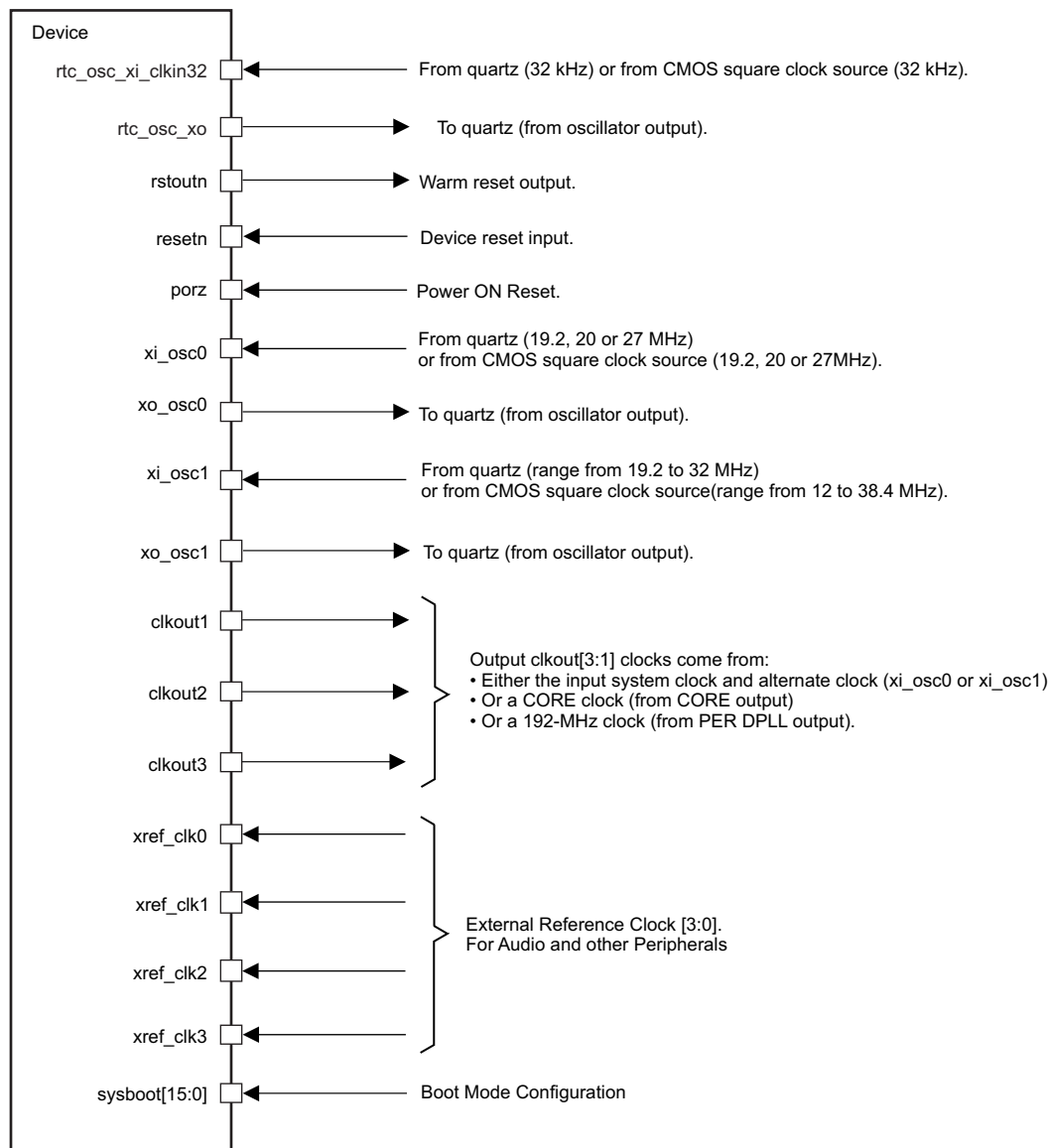
图 6-1. Clock Interface
