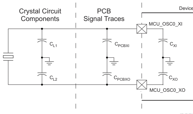
图 7-19. Load Capacitance
