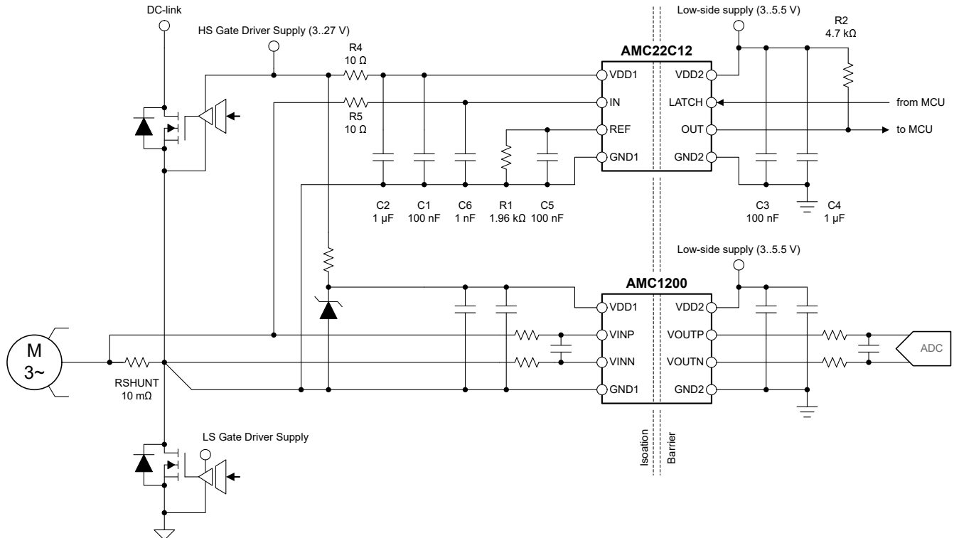
图 8-1. 使用 AMC22C12 进行过流检测
