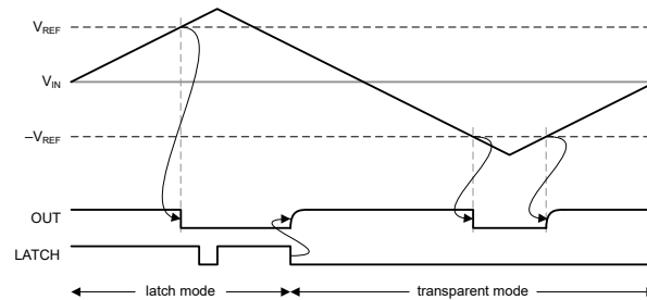
图 6-2. 功能时序图
