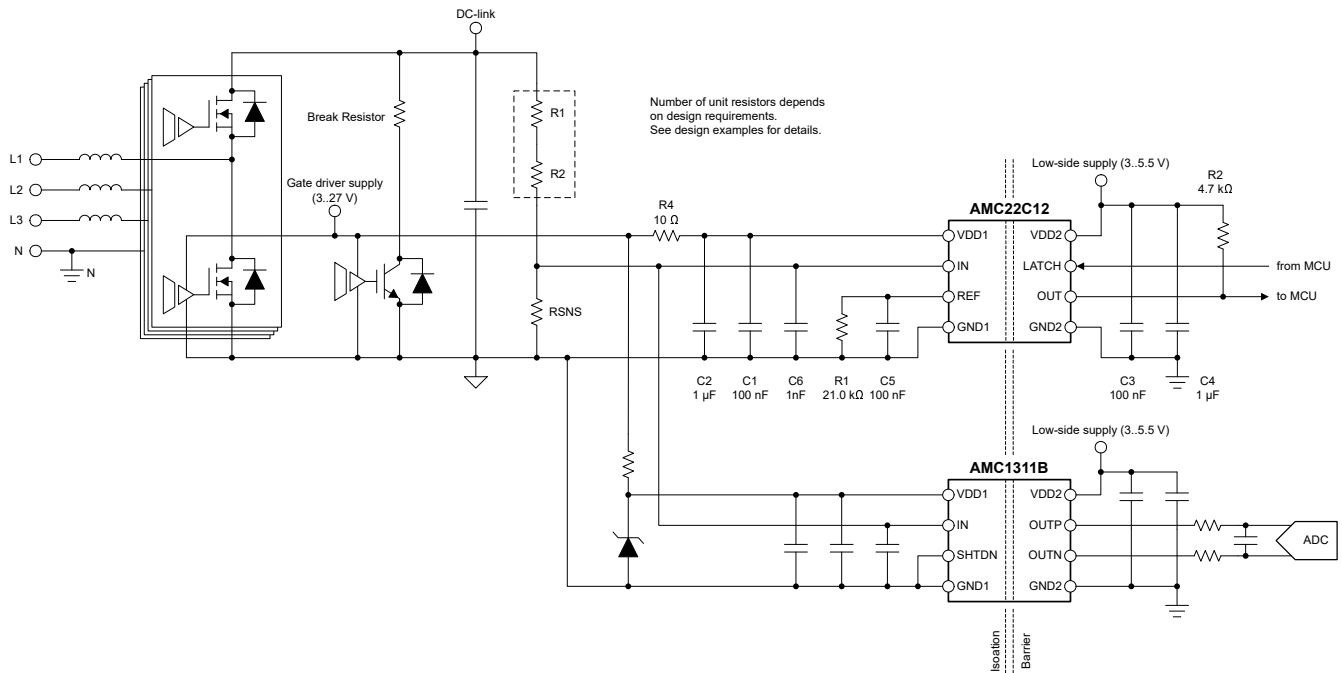
图 8-2. 使用 AMC22C12 进行过压检测
