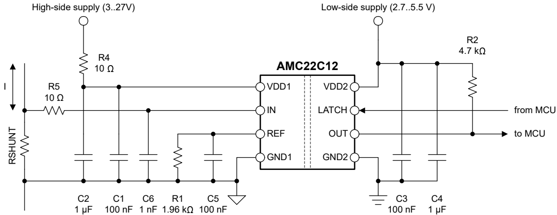
图 9-1. 去耦 AMC22C12
