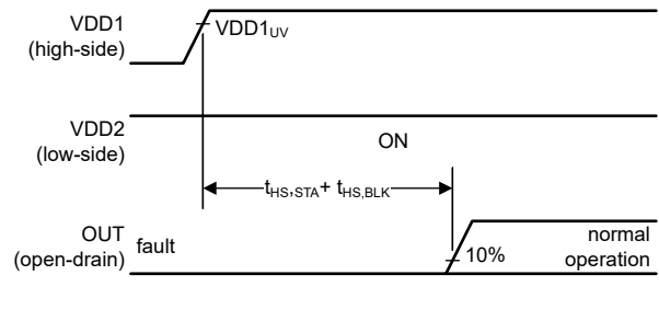
图 7-6. VDD2 保持开启; VDD1 开启 (长延迟)
