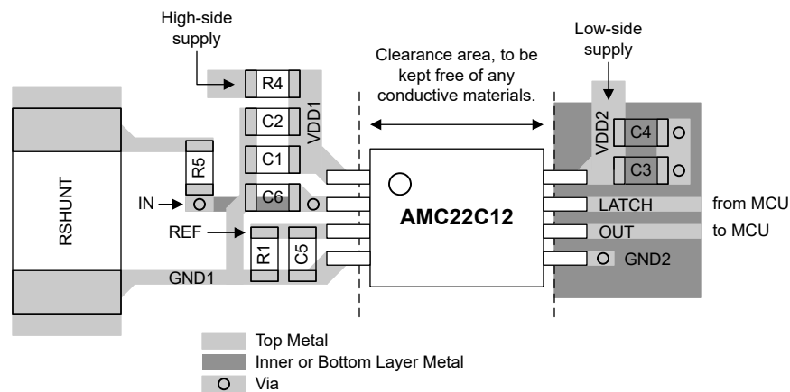
图 10-1. 建议布局 AMC22C12
