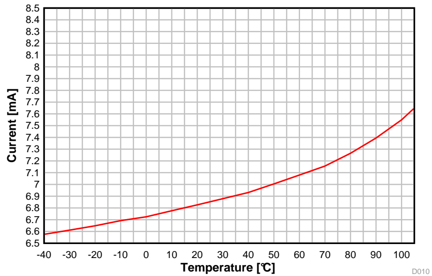
图 5-7. RX Current vs. Temperature (BLE 1 Mbps, 2.44 GHz)
