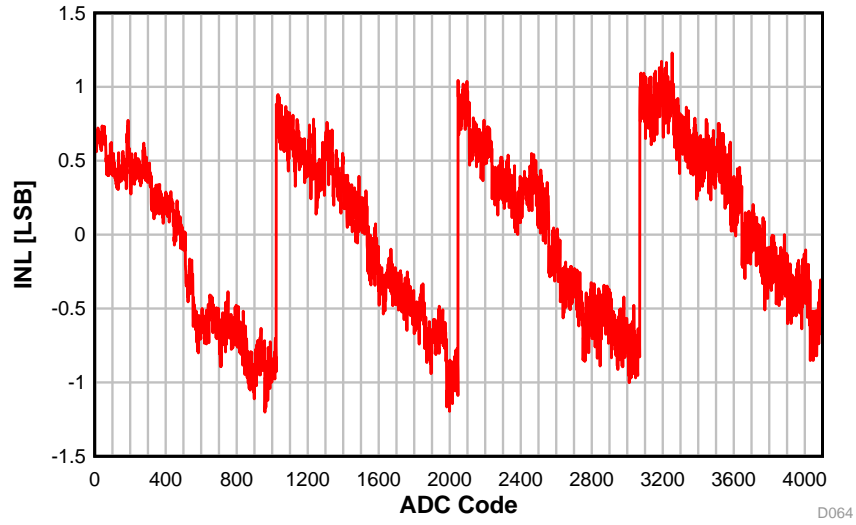
图 5-23. INL vs. ADC Code
