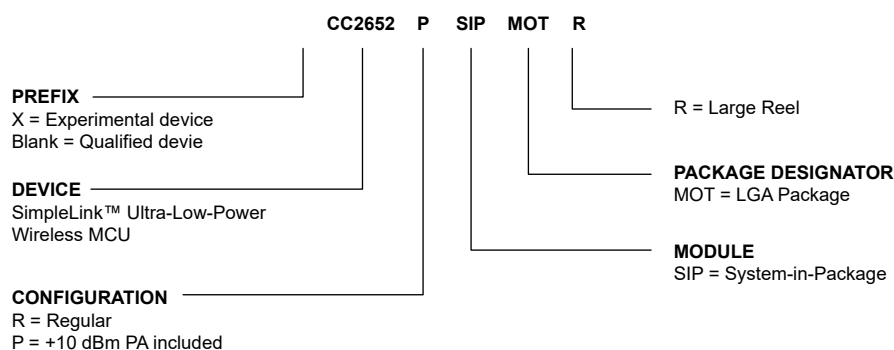
图 12-1. Device Nomenclature
