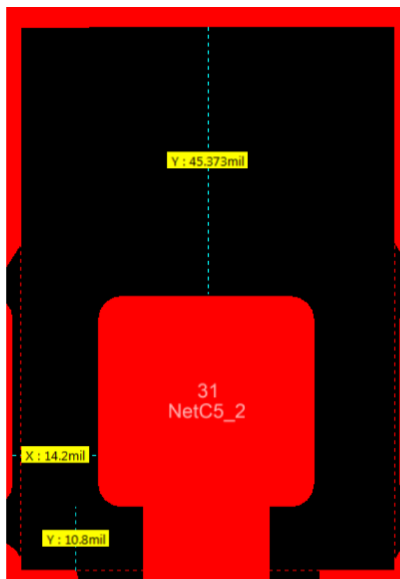
图 10-6. Top Layer Copper Pullback on RF Pads
