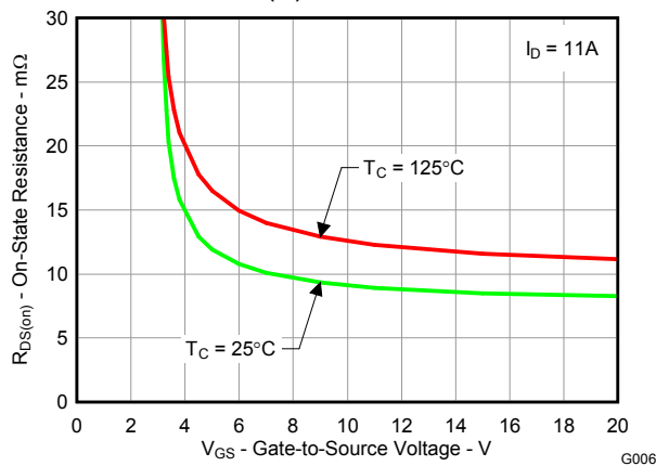
R_{DS(on)} 与 V_{GS} 的关系曲线
