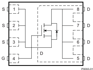
顶视图
