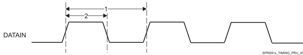
图 5-113. PRU-ICSS PRU Shift In Timing
