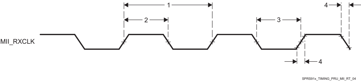
图 5-125. PRU-ICSS MII[x]_RXCLK Timing
