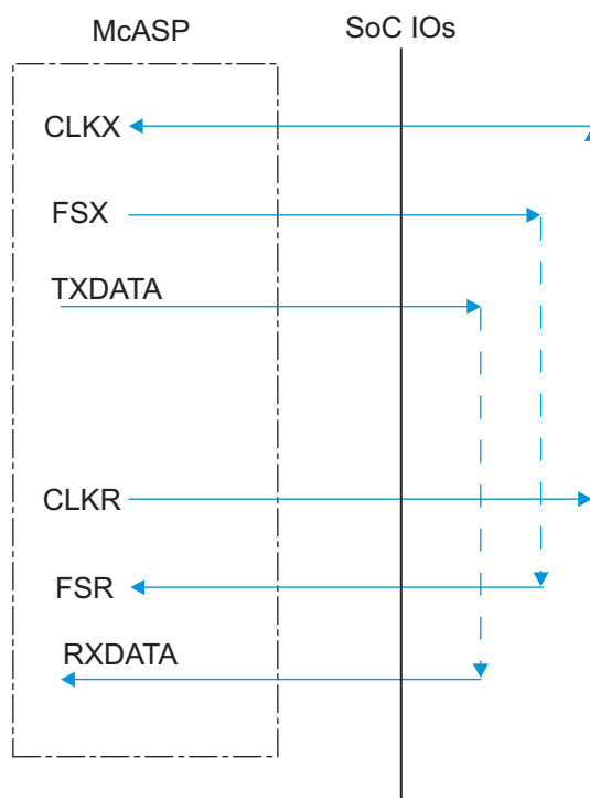
图 5-62. McASP1-8 CIOFOI – ASYNC Mode
