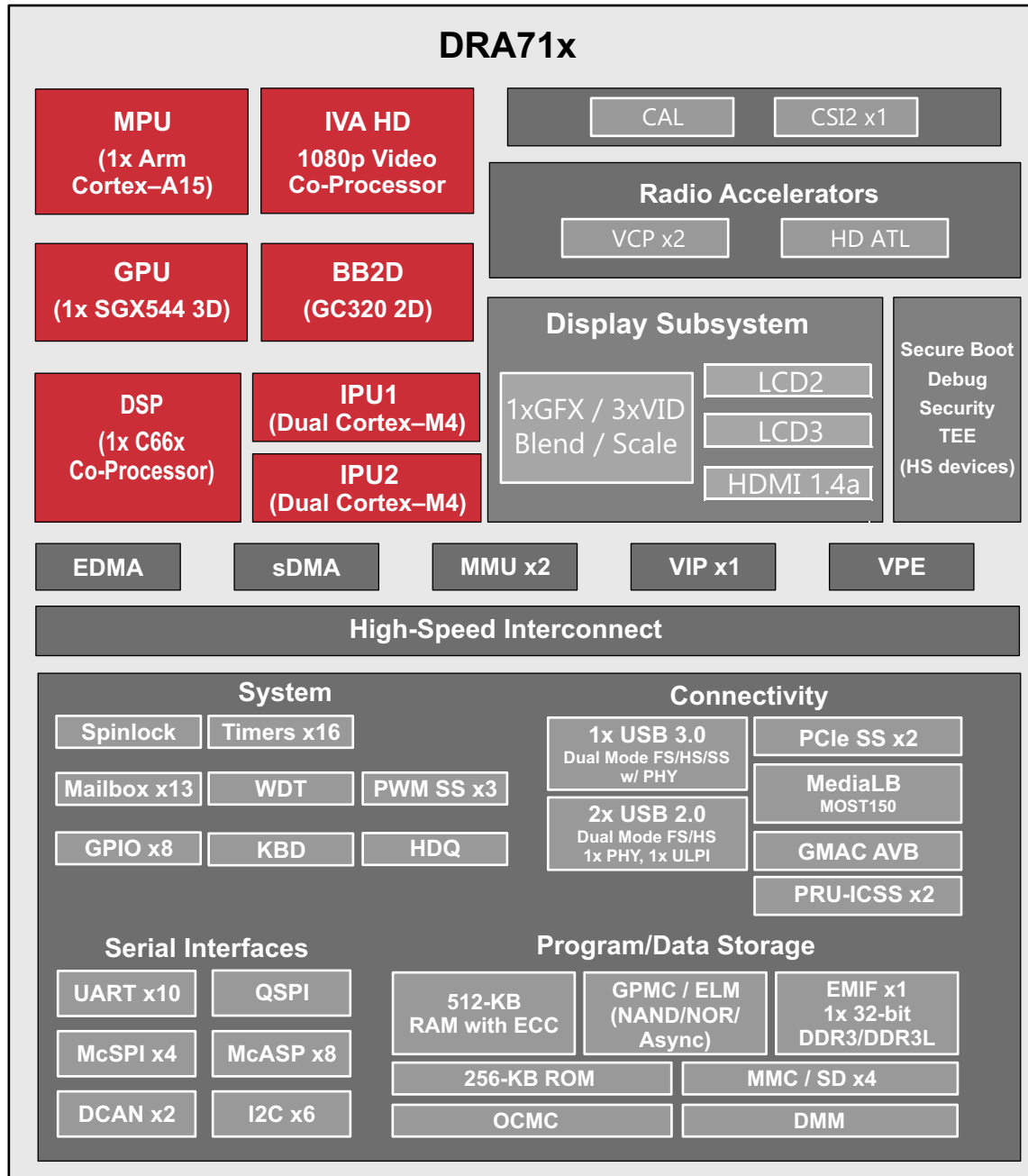
图 1-1. DRA71x 方框图
