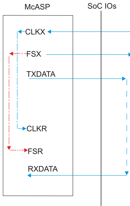
图 5-64. McASP1-8 CI-FO- – SYNC Mode
