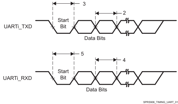
图 5-48. UART Timing
