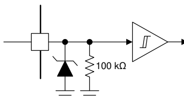
图 9-9. Logic-level input
