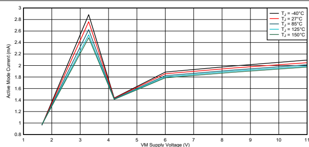
图 8-1. Active Mode Current
