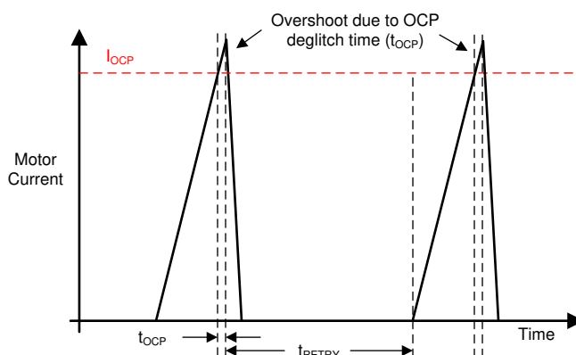
图 9-6. OCP Operation
