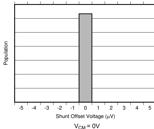
图 6-3. 分流输入失调电压产生分布图
