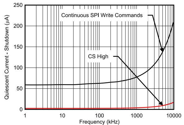
图 6-23. 关断 I_Q 与时钟频率间的关系
