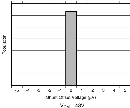
图 6-2. 分流输入失调电压产生分布图
