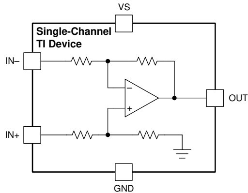
图 8-1. INA180-Q1 Functional Block Diagram
