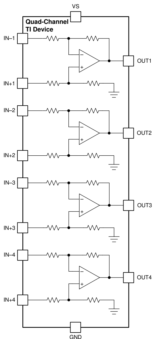
图 8-3. INA4180-Q1 Functional Block Diagram
