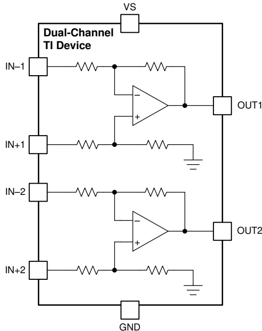
图 8-2. INA2180-Q1 Functional Block Diagram
