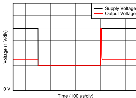
图 7-36. Brownout Recovery
