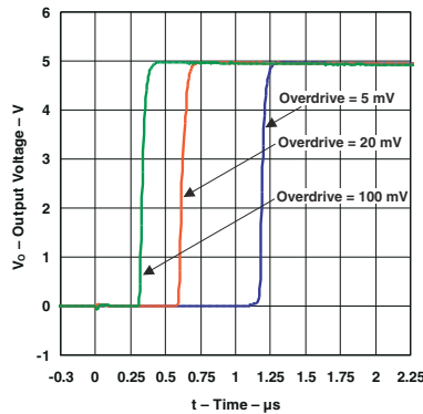
图 6-5. 正转换时各种过驱的响应时间
