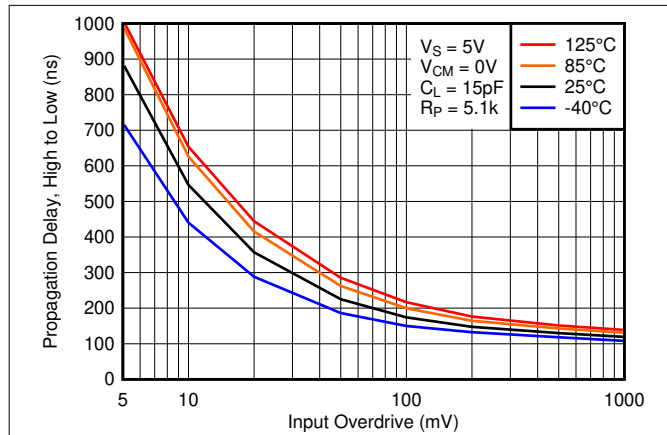
图 6-30. 高电平至低电平传播延迟与输入过驱电压之间的关系, 5V
