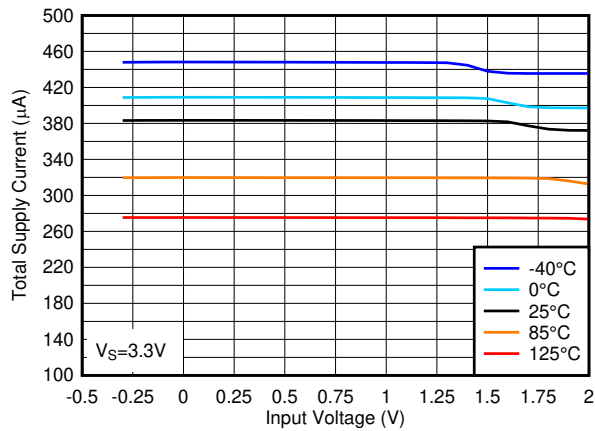
图 6-8. 3.3V 下总电源电流与输入电压之间的关系
