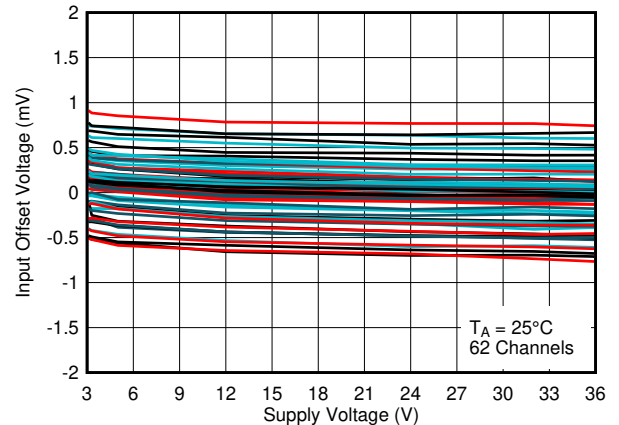
图 6-17. 25°C 下输入失调电压与电源电压之间的关系
