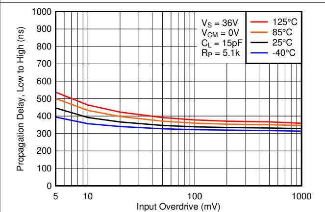
图 6-35. 低电平至高电平传播延迟与输入过驱电压之间的关系, 36V
