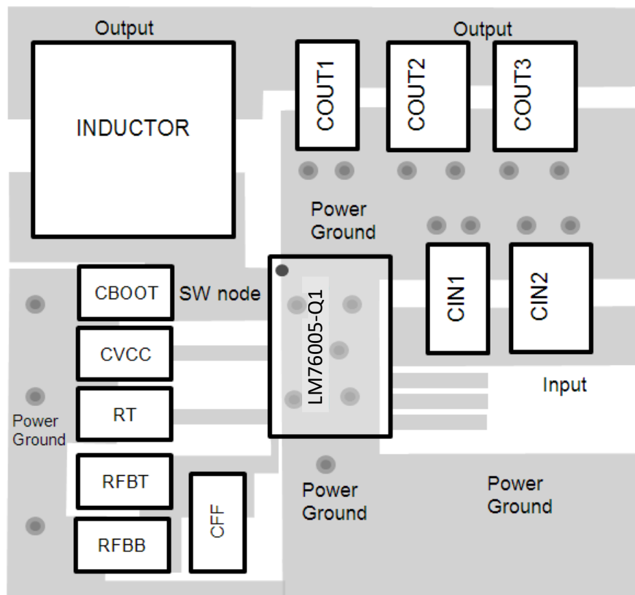
图 10-3. LM76005-Q1 Layout
