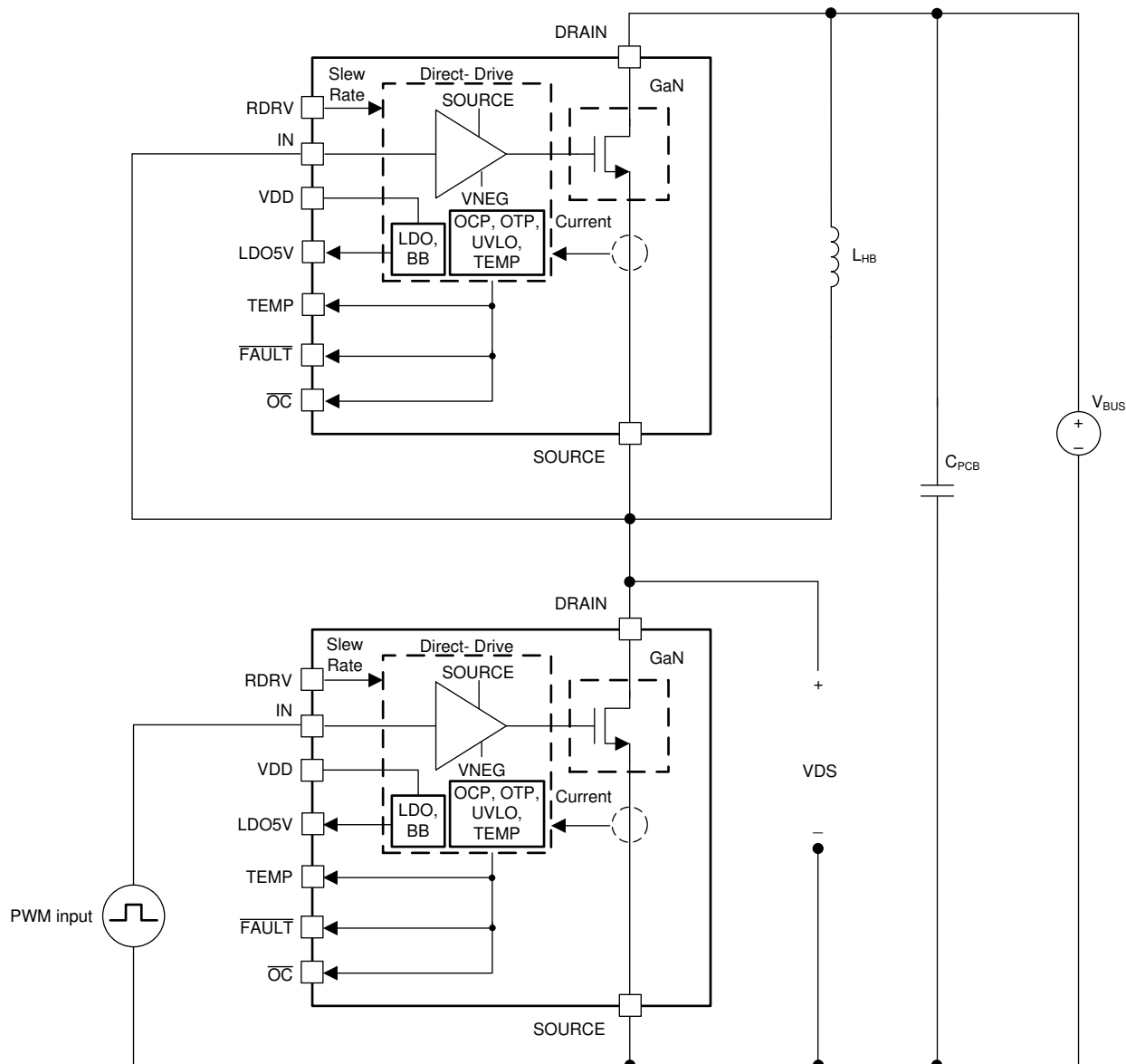
图 8-1. 电路用于确定开关参数
