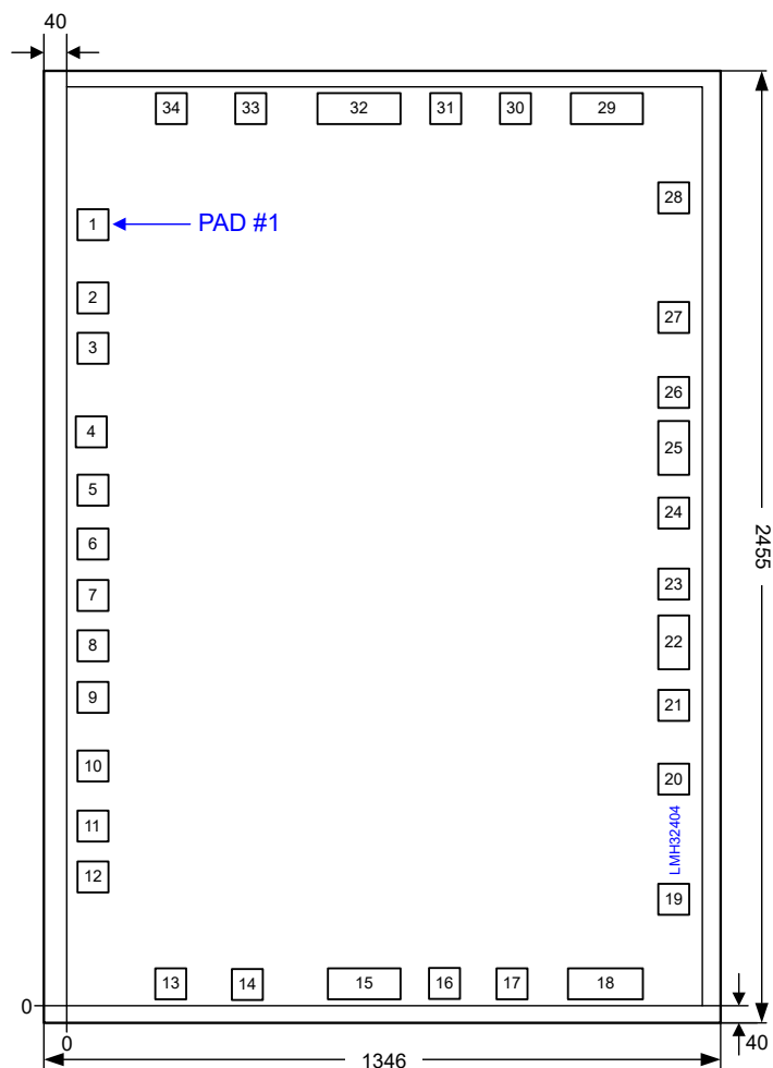
图 5-2. Bare Die Package (Preview)
