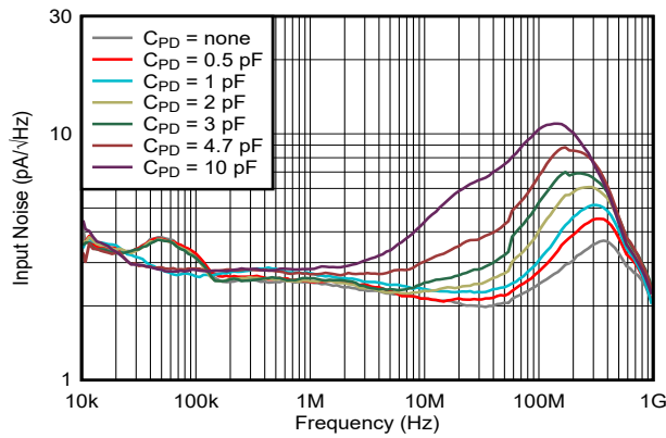
图 6-7. Input Noise Density vs Input Capacitance
