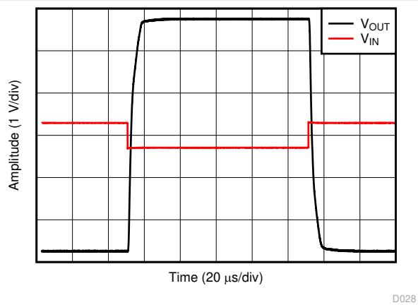
图 6-23. 过载恢复
