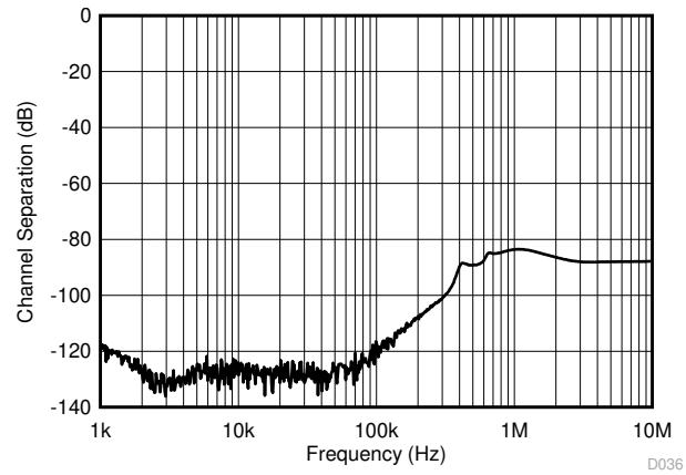
图 6-31. 通道分离
