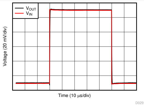
图 6-22. 无相位反转
