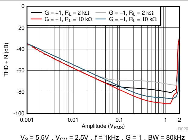
图 6-15. THD + N 与幅度间的关系
