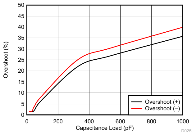
图 6-20. 小信号过冲与容性负载间的关系
