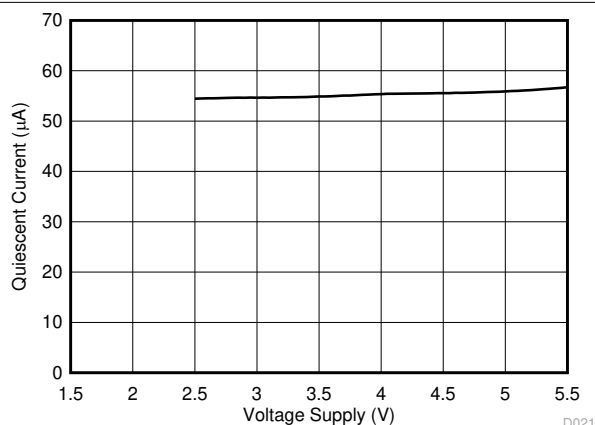
图 6-16. 静态电流与电源电压间的关系
