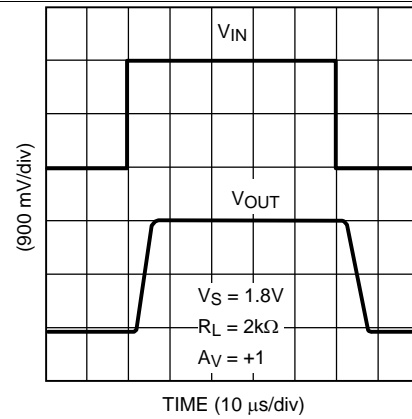
Figure 24. 大信号同相响应
