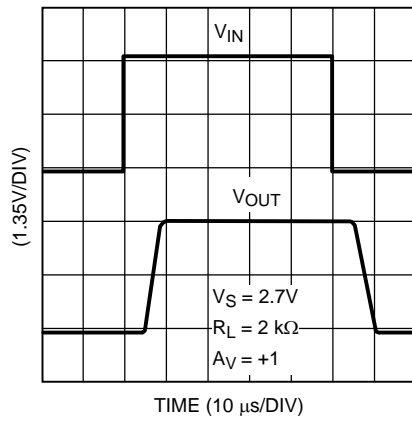
Figure 25. 大信号同相应
