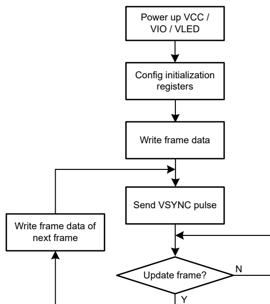
图 9-3. Program Procedure
