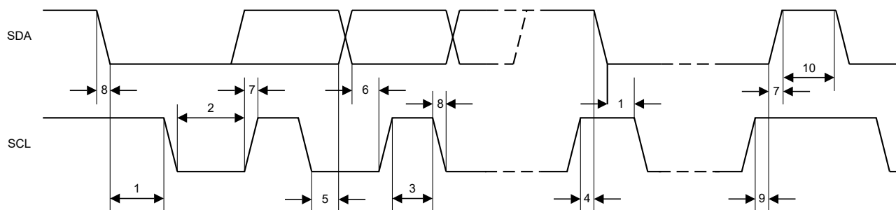
图 7-2. I 2 C Timing Parameters
