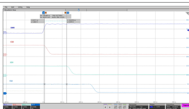
图 9-5. PWM Phase Shift Enabled
