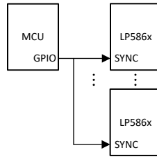
图 8-6. Multiple Devices Sync
