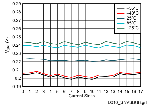
图 7-8. V_{SAT} vs Current Sinks (10 mA)
