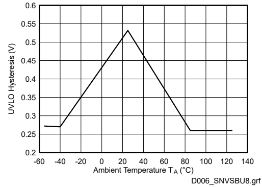
图 7-4. V_{CC} UVLO Hysteresis
