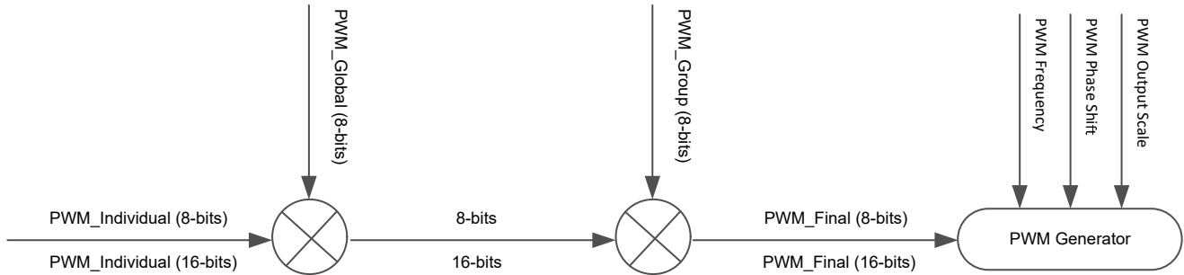
图 8-3. PWM Control Scheme
