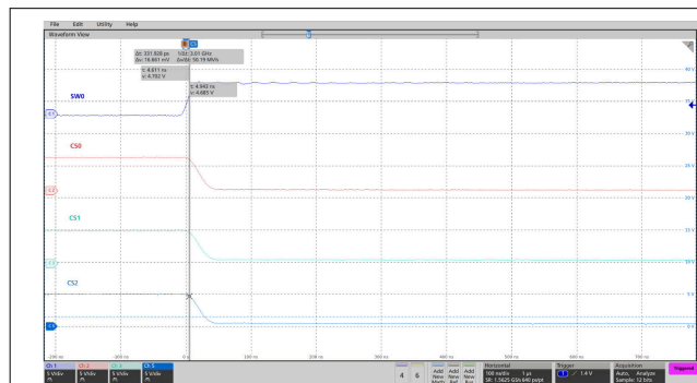
图 9-4. PWM Phase Shift Disabled
