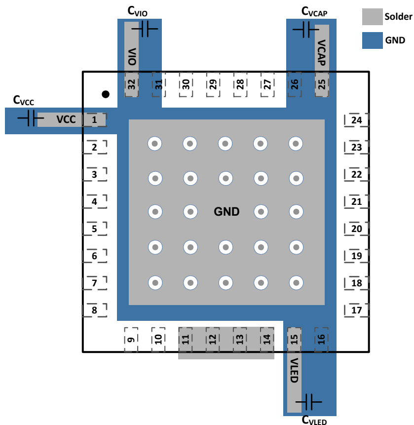
图 11-1. LP5861 Layout Example
