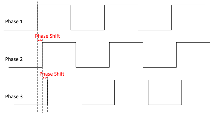
图 8-1. Phase Shift
