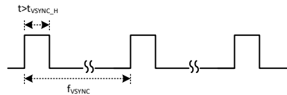
图 8-7. VSYNC Timing
