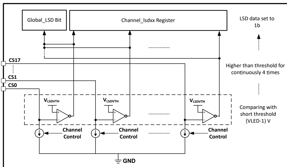
图 8-9. LSD Circuit
