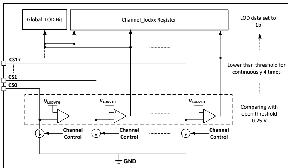
图 8-8. LOD Circuits
