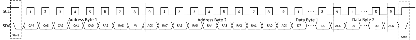
图 8-11. I²C Write Timing
