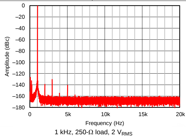
图 46. Output Spectrum
