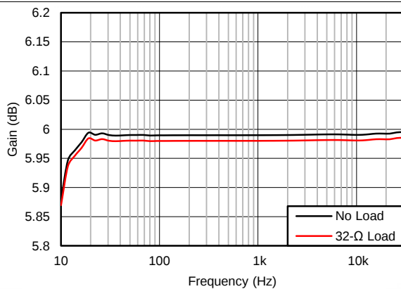
图 42. Amplifier Transfer Function
