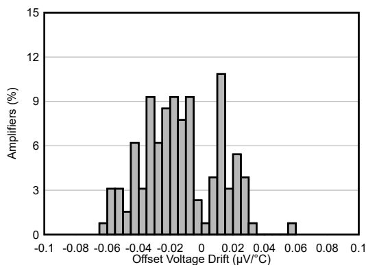
OPAx205 失调电压漂移
