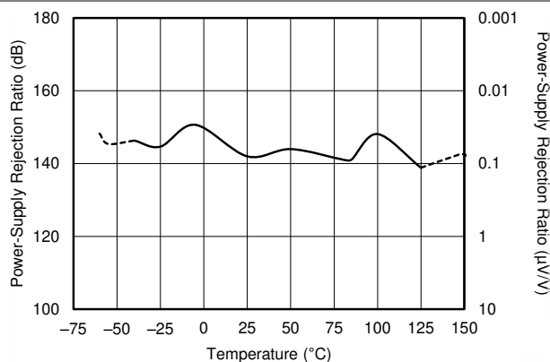
图 6-14. PSRR vs Temperature
