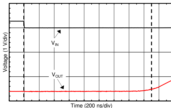
图 6-26. No Phase Reversal
