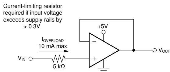
图 7-3. Input Current Protection
