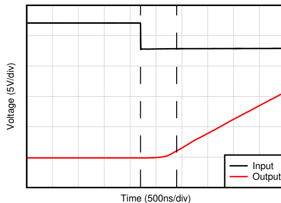
图 6-38. 负过载恢复
