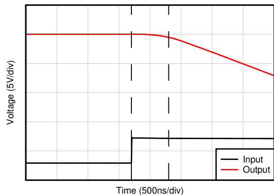
图 6-37. 正过载恢复
