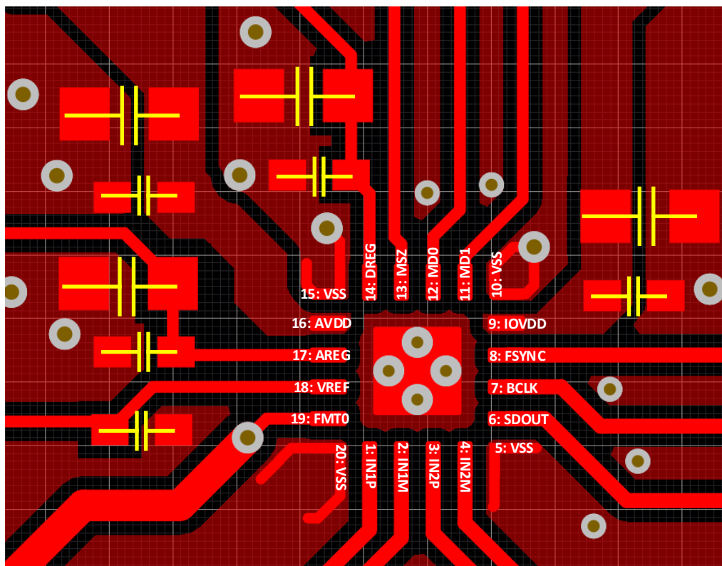
图 11-1. Example Layout
