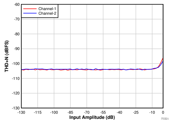
图 9-7. PCM1821: THD+N vs Input Amplitude
