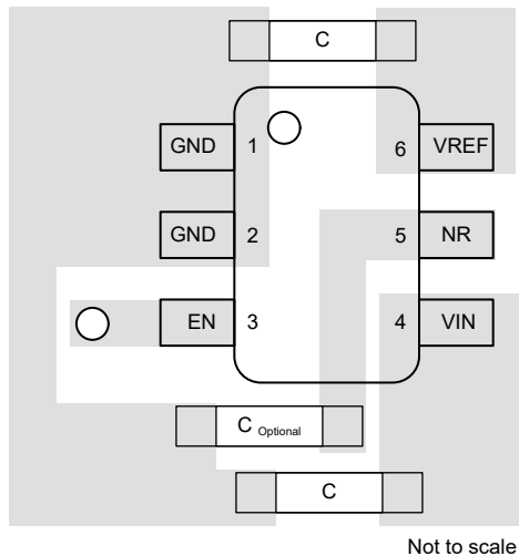
图 10-4. Layout Example
