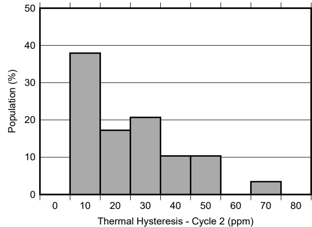
图 8-9. Thermal Hysteresis Distribution - 40°C to 105°C, Cycle 2
