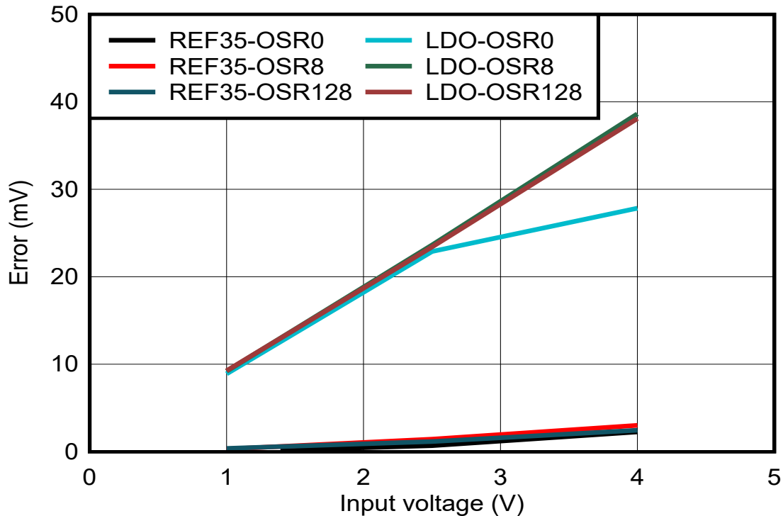
图 10-3. Error vs Input Voltage
