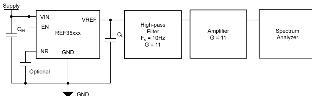
图 8-14. Broadband Noise Test Setup
