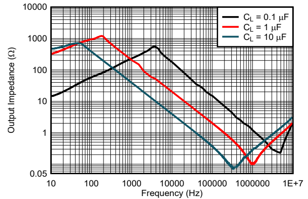
图 7-26. Output Impedance
