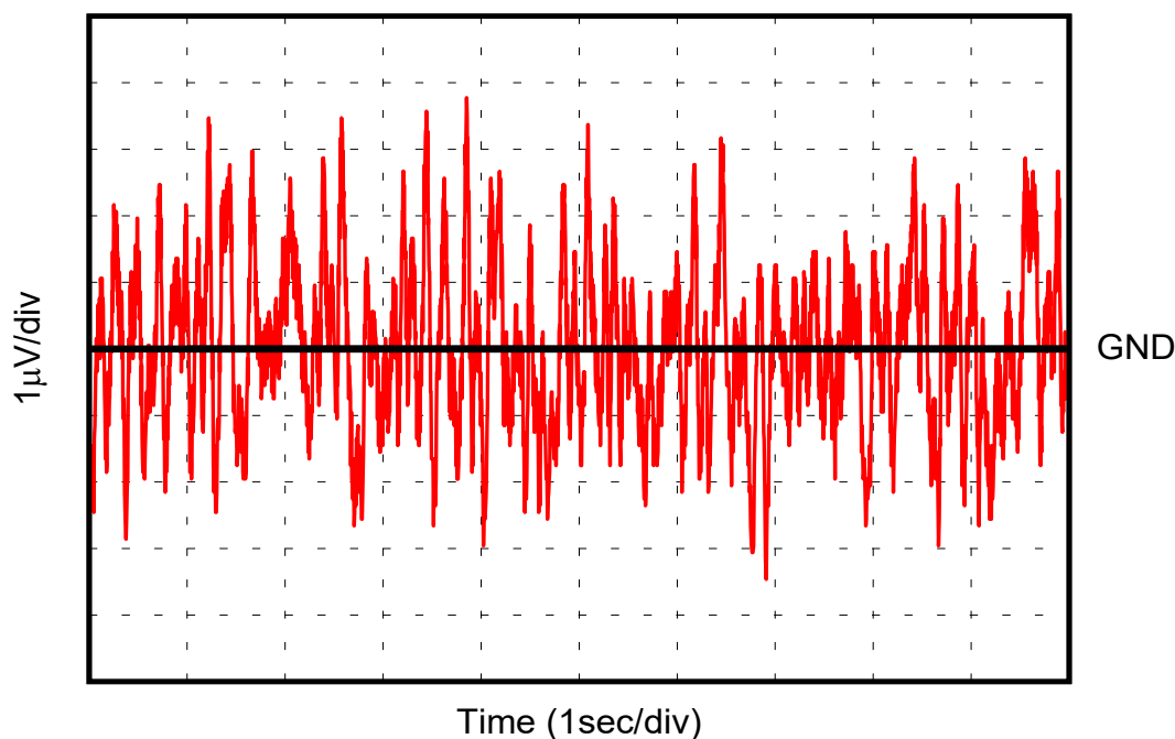
图 8-11. 0.1 Hz to 10 Hz Voltage Noise
