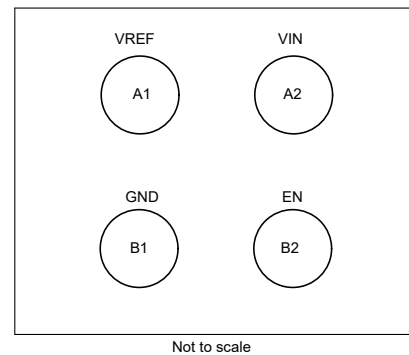
图 6-2. YBH Package 4-Pin WCSP Top View
