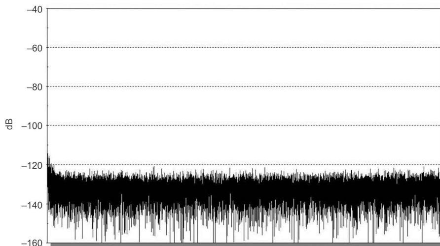
图 10-2. 数据采集系统的本底噪声 FFT 图
