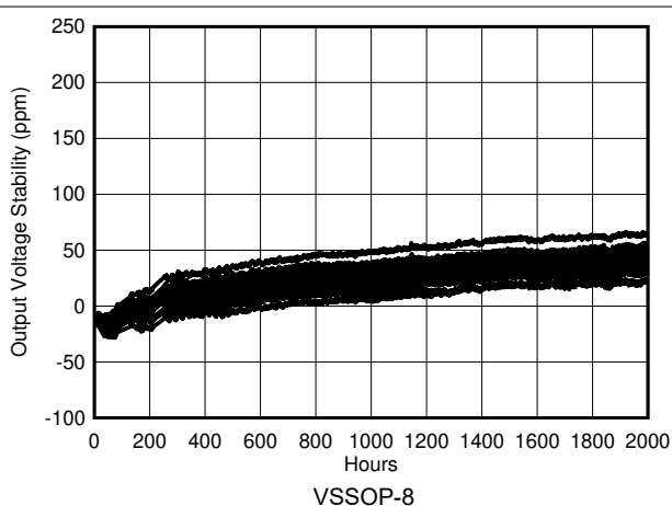
图 7-24. REF50xx 长期稳定性 (前 2000 小时)
