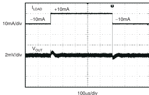
图 7-19. 负载瞬态
