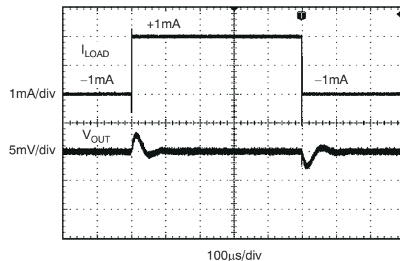
图 7-16. 负载瞬态
