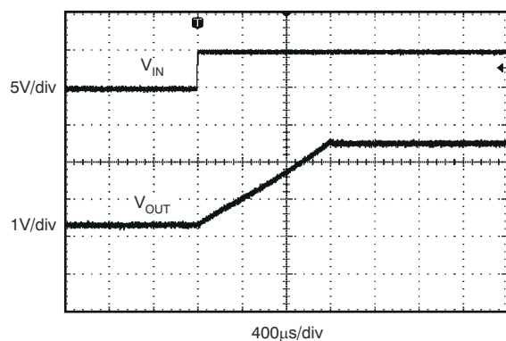
图 7-15. 启动
