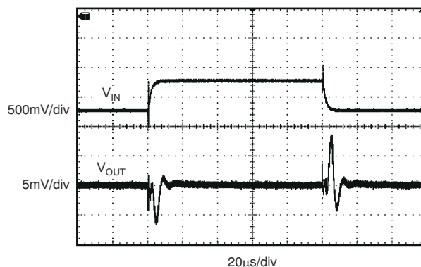
图 7-20. 线路瞬态
