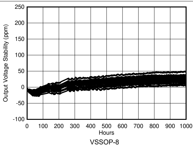
图 7-22. REF50xx 长期稳定性 (前 1000 小时)
