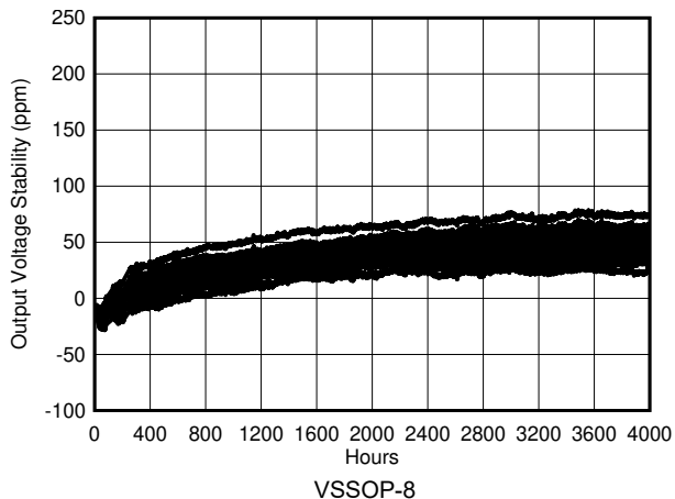
图 7-26. REF50xx 长期稳定性 ( 4000 小时 )
