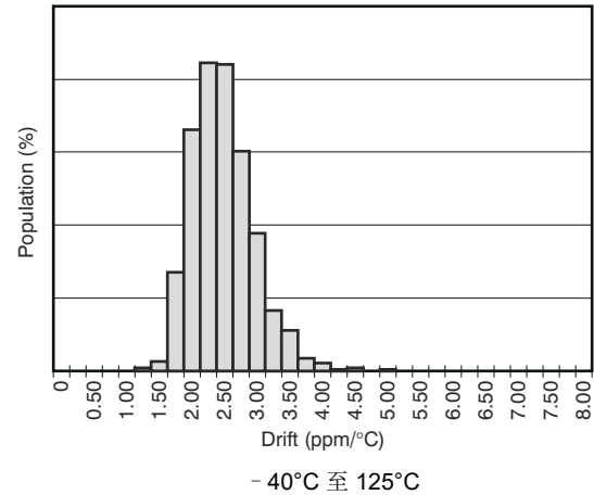
图 7-2. 温漂
