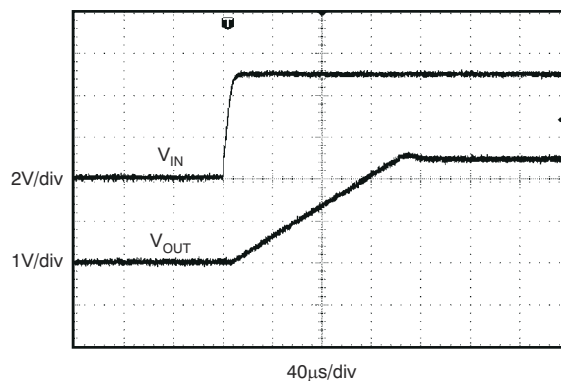
图 7-14. 启动
