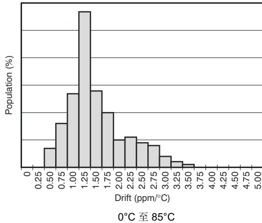
图 7-1. 温漂
