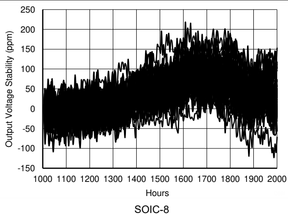
图 7-28. REF50xx 长期稳定性 ( 后 1000 小时 )
