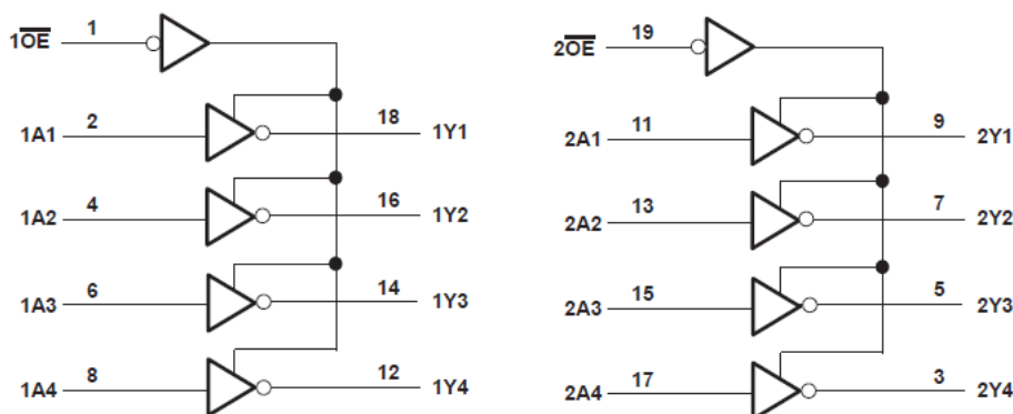
功能方框图
