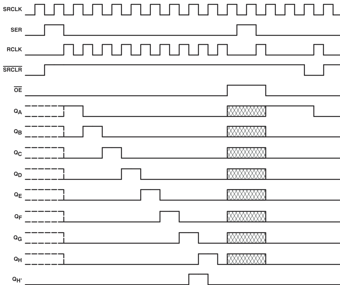
图 6-1. 时序图
