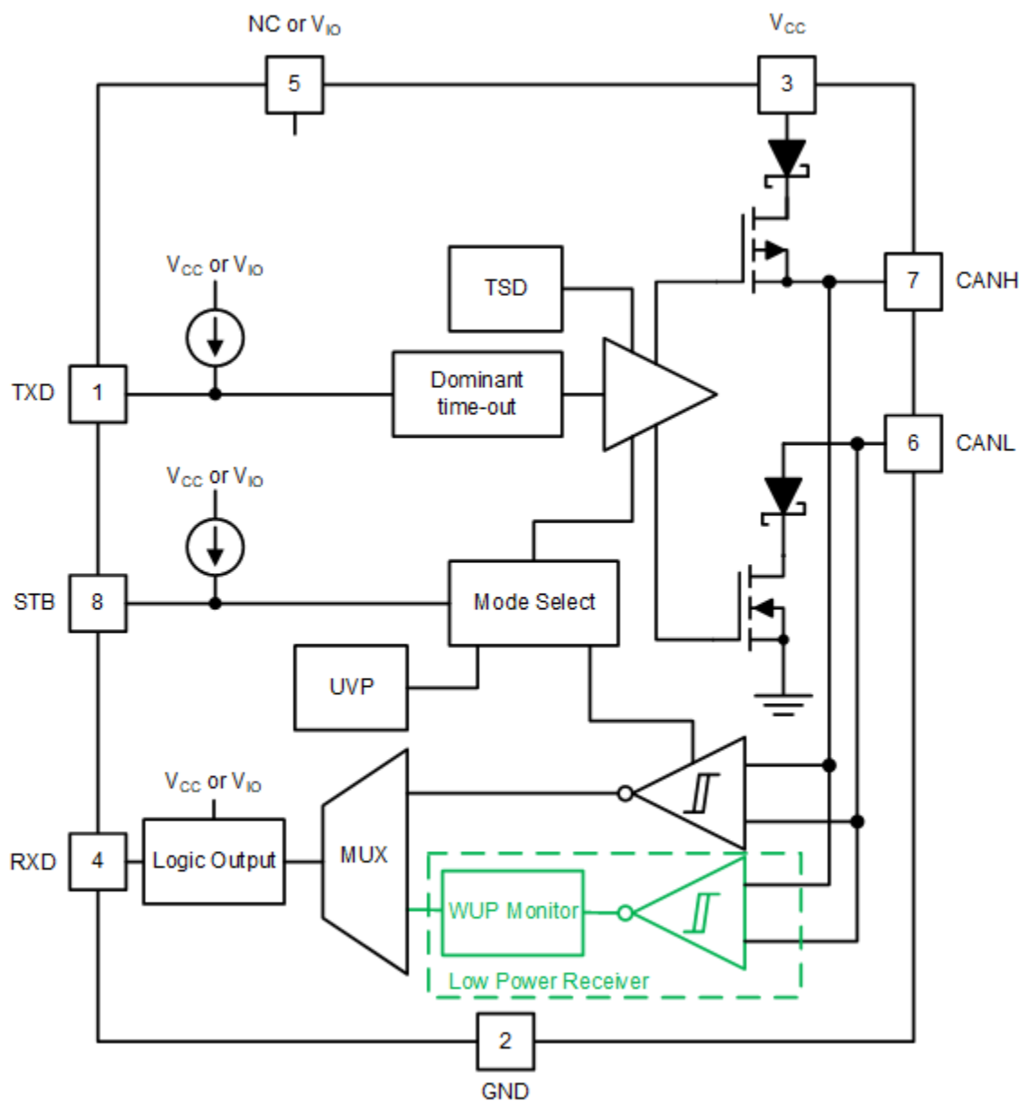
图 9-1. Block Diagram
