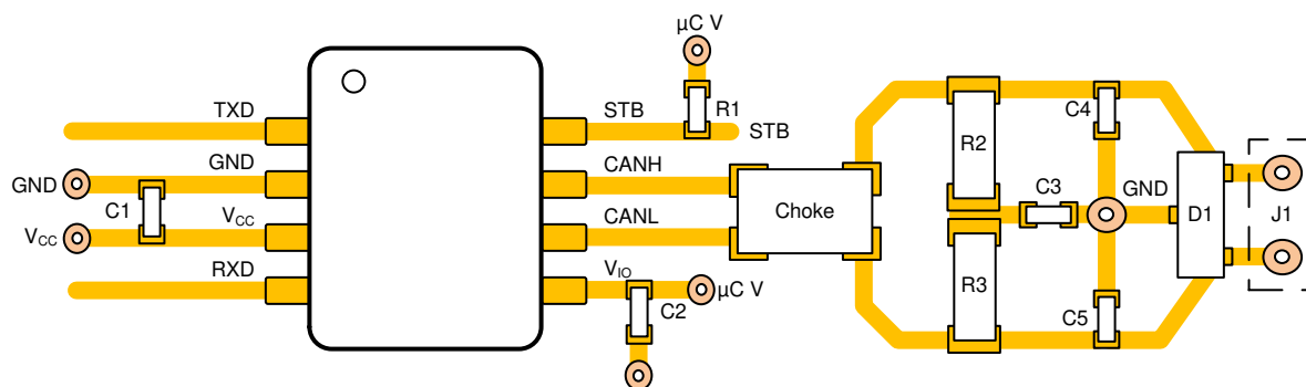
图 12-1. Layout Example
