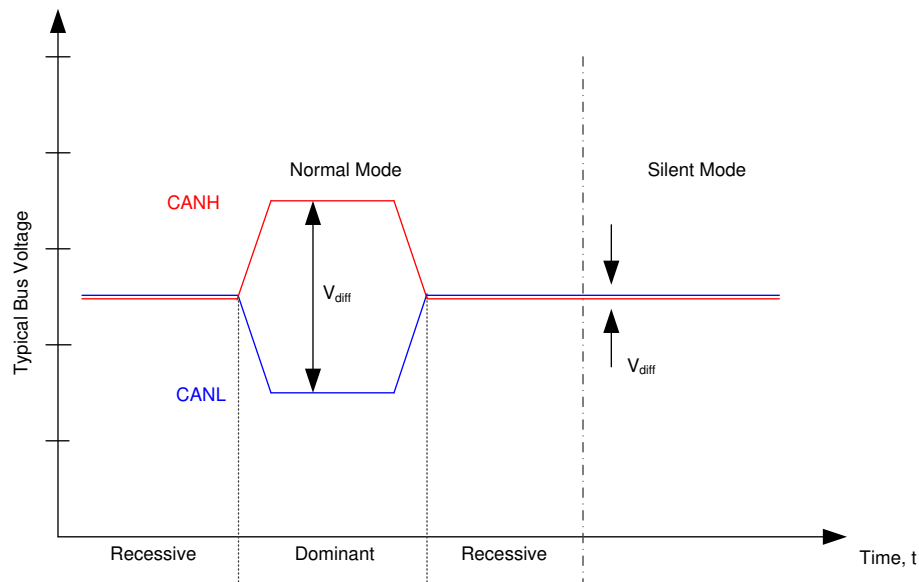
图 8-1. Bus States
