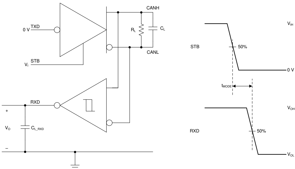
图 9-5. t_{\text{MODE}} 测试电路与测量
