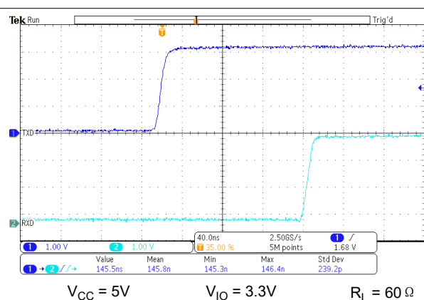
图 11-5. t_{PROP(LOOP2)}
