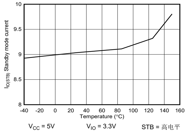
图 8-4. I_{IO(standby)} 与温度间的关系
