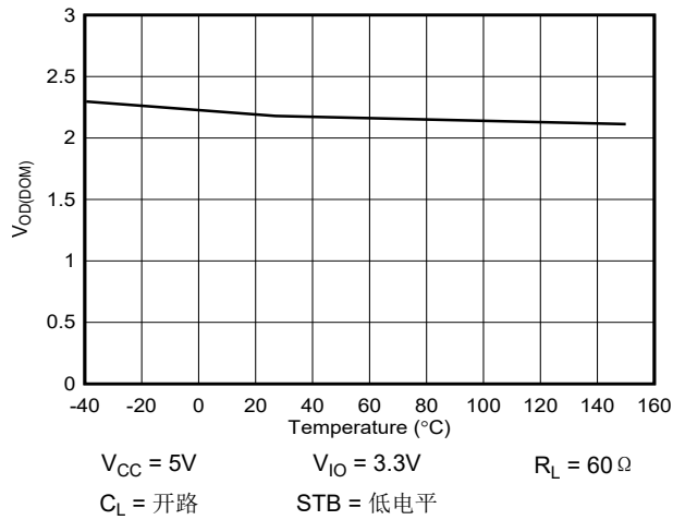
图 8-1. V_{OD(DOM)} 过热
