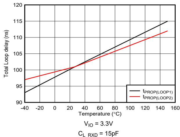
图 8-5. 总环路延迟 t_{PROP(LOOP1)} 和 t_{PROP(LOOP2)} 与温度间的关系
