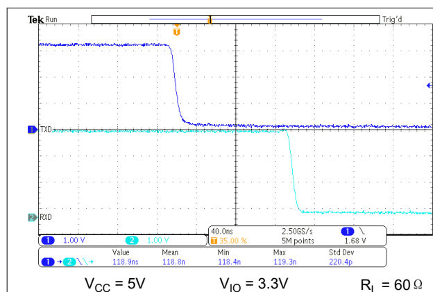
图 11-4. t_{PROP(LOOP1)}
