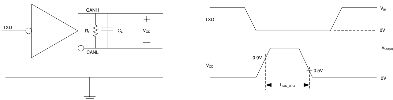
图 9-6. TXD 显性超时测试电路与测量
