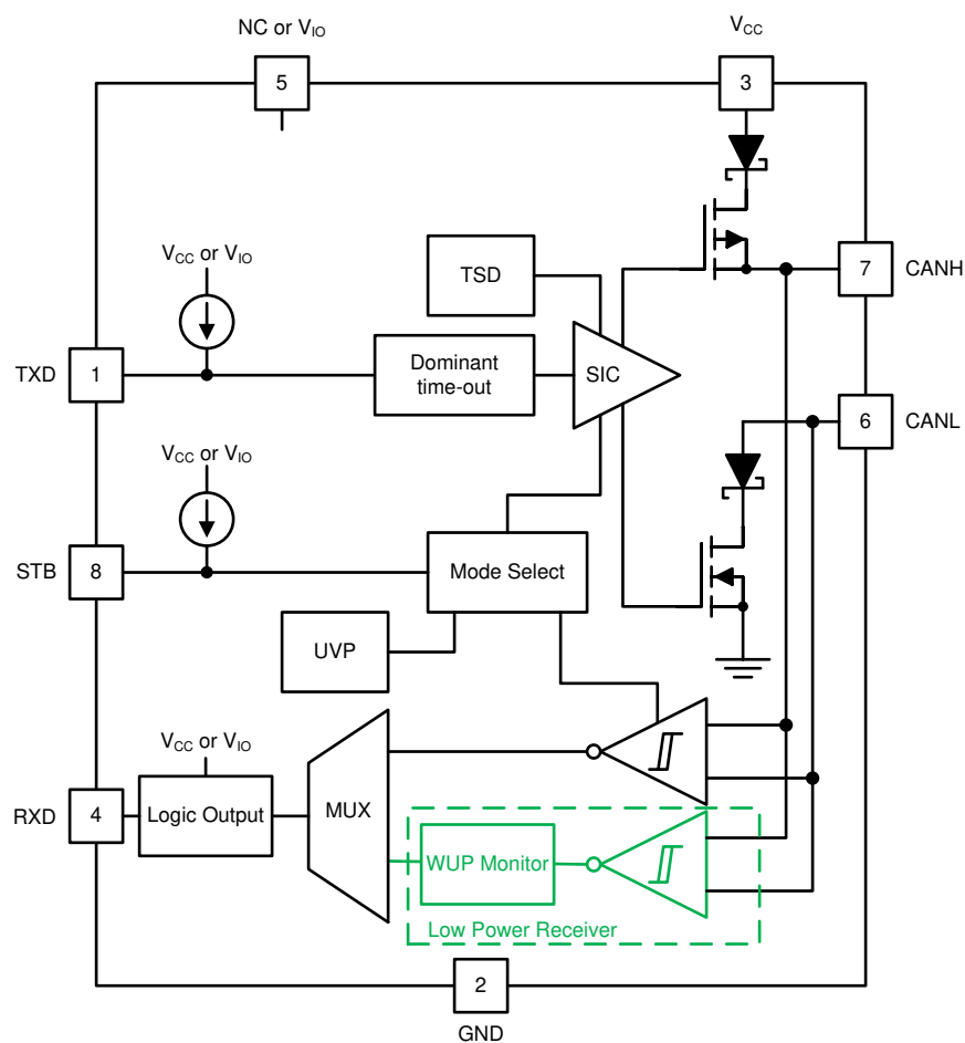
图 10-3. 方框图
