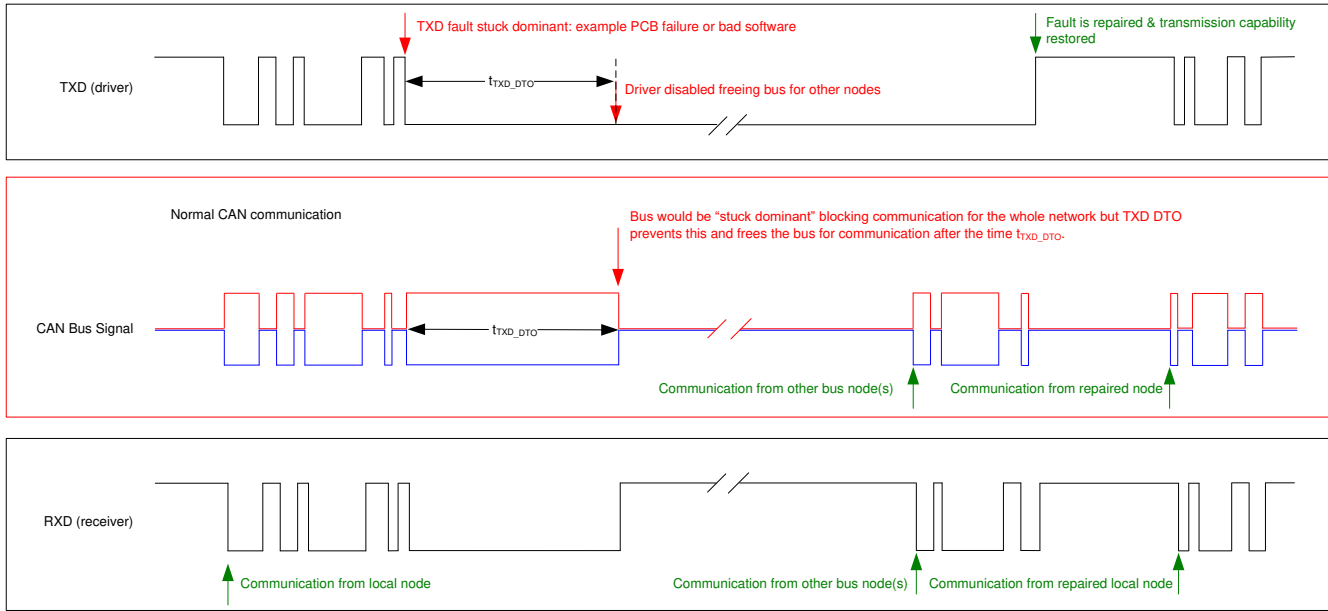
图 10-6. TXD 显性超时的时序图示例
