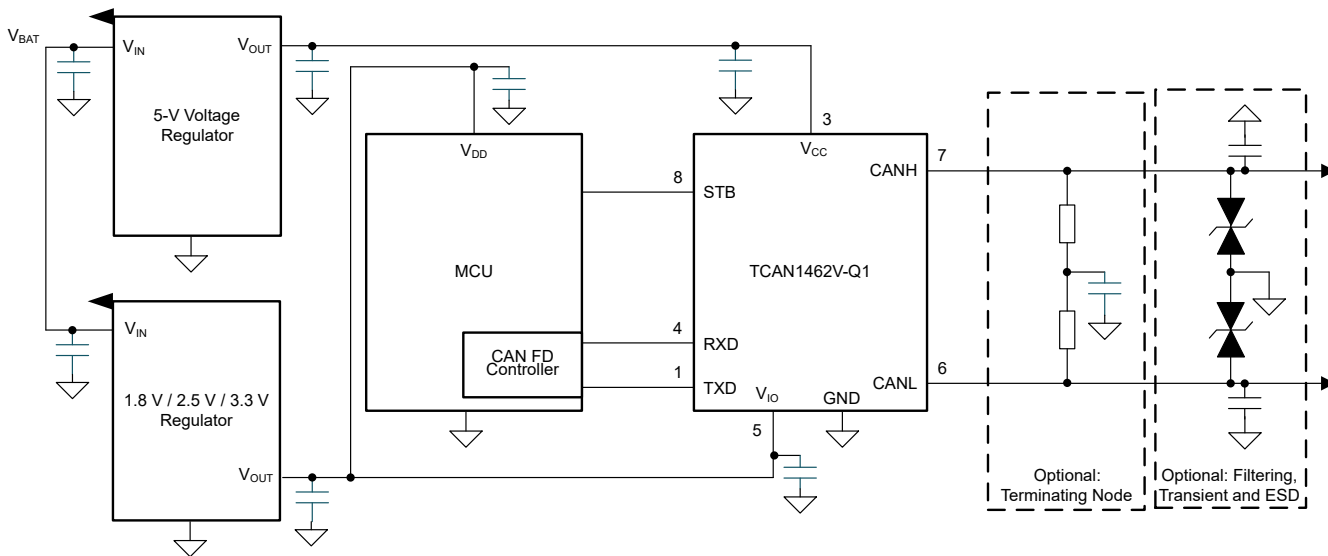
图 11-6. 使用 1.8V、2.5V、3.3V IO 连接的典型收发器应用
