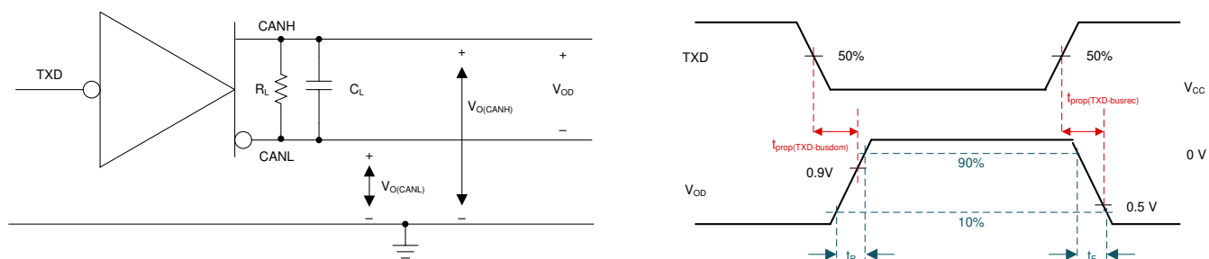
图 9-2. 驱动器测试电路与测量
