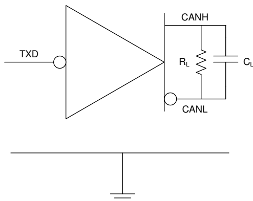
图 9-1. I_{CC} 测试电路
