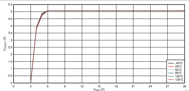
图 9-9. V_{CCOUT} vs V_{SUP}
