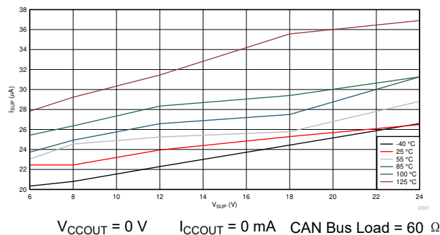
图 6-1. I_{SUP} vs V_{SUP} Sleep Mode
