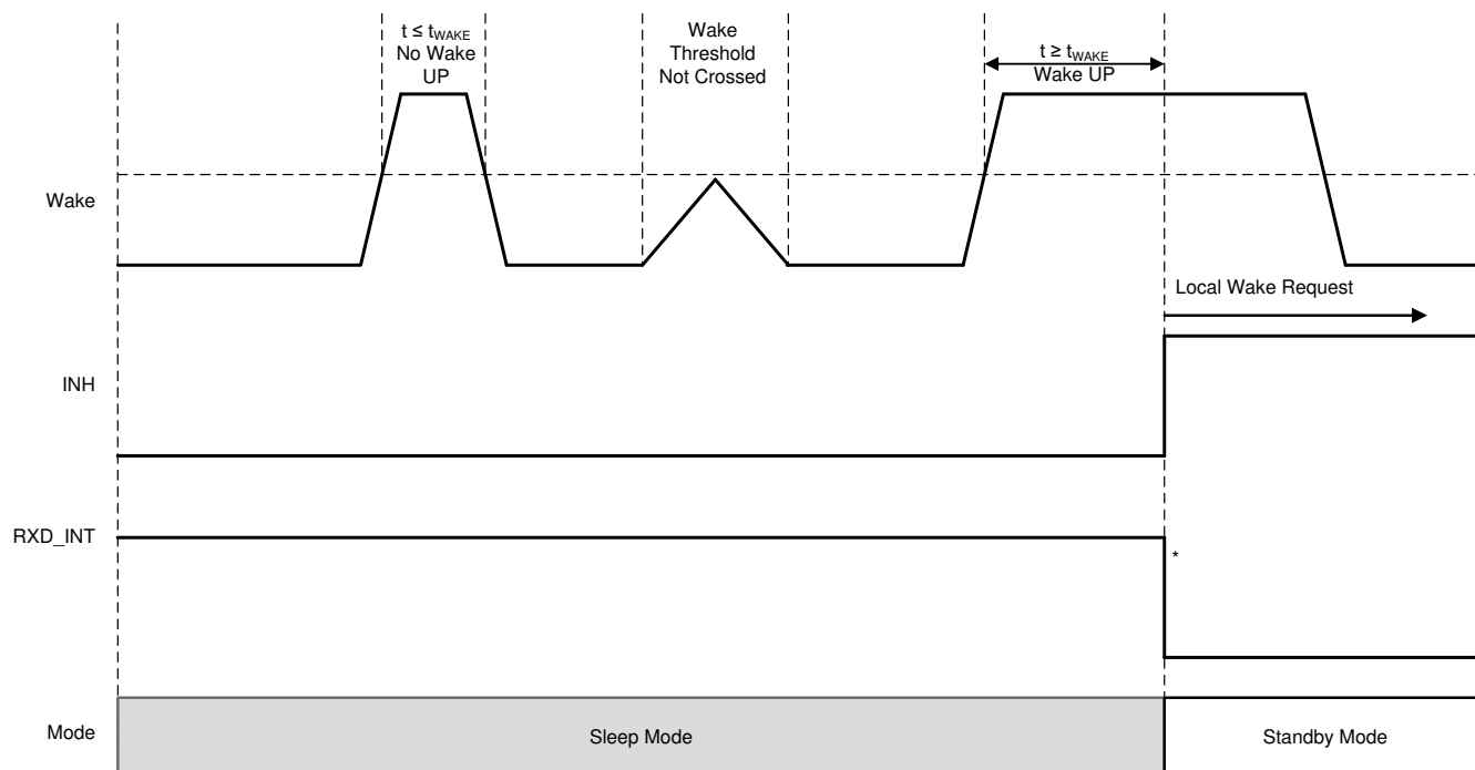
图 8-8. Local Wake-Up: Rising Edge
