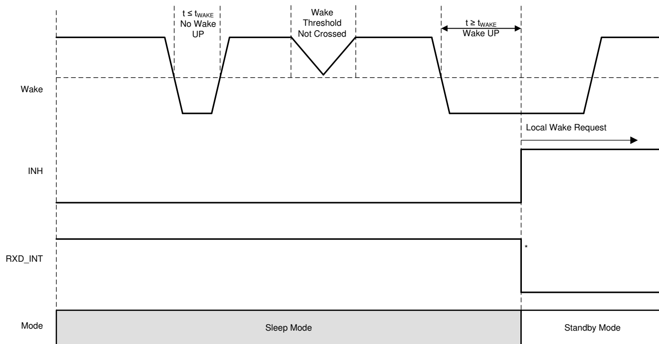
图 8-9. Local Wake-Up: Falling Edge
