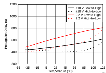
稳定传播延迟与温度
