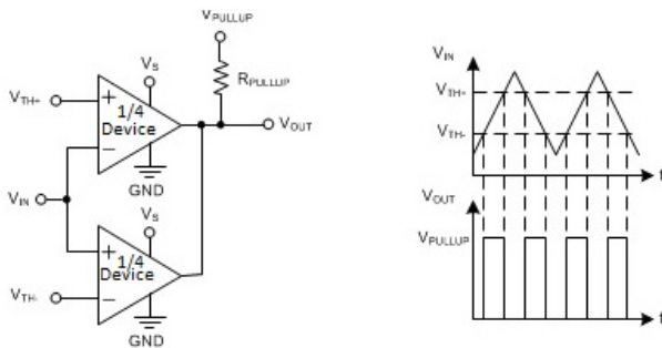
TLV1704-SEP 用作窗口比较器
