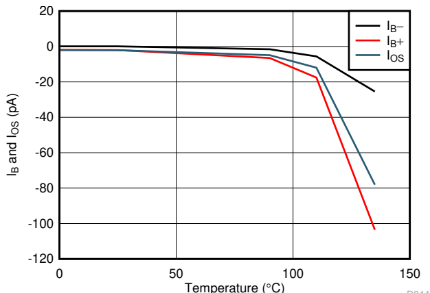
图 7-8. I_B 和 I_{OS} 与温度间的关系
