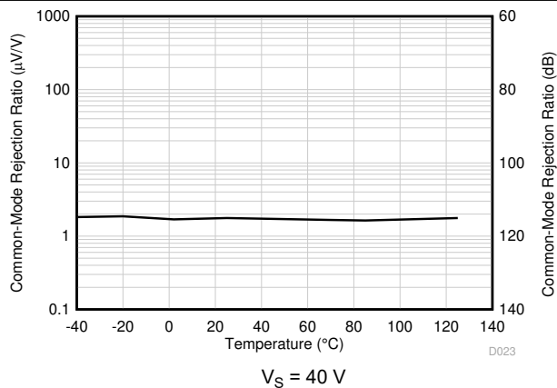
图 6-17. CMRR vs Temperature
