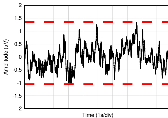
图 6-20. 0.1-Hz to 10-Hz Noise
