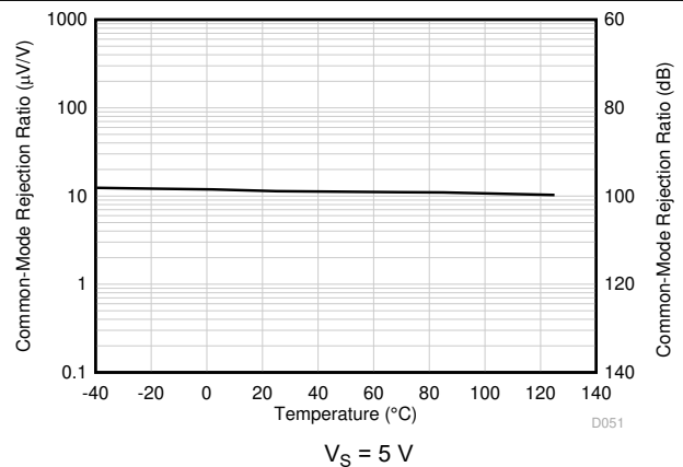
图 6-18. CMRR vs Temperature
