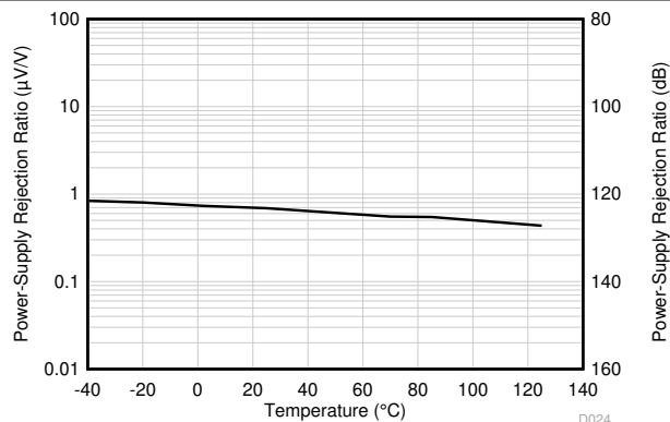
图 6-19. PSRR vs Temperature
