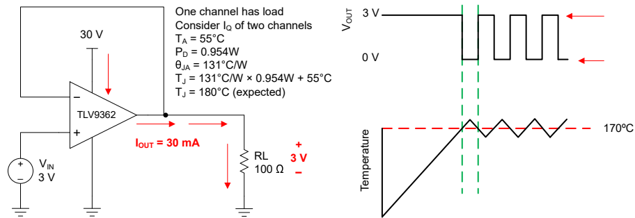
图 7-2. Thermal Protection
