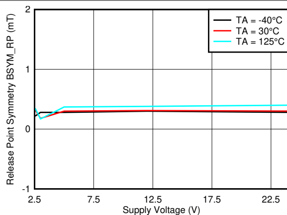
图 7-31. B_{SYM\_RP(ZY)} vs. V_{CC}
