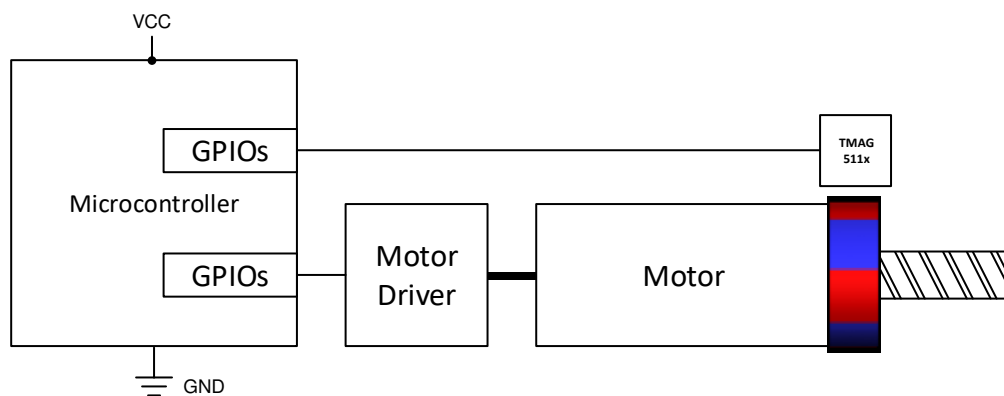
图 9-1. Incremental Encoding
