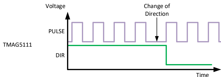
图 9-3. TMAG5111-Q1 Output Response
