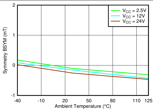
图 7-60. B_{SYM(X)} vs. Temperature
