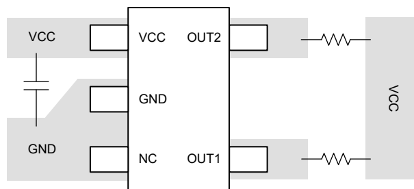
图 11-1. Layout Example
