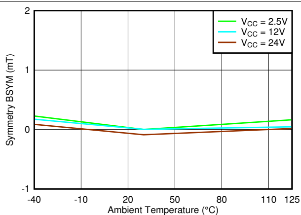
图 7-62. B_{SYM(Y)} vs. Temperature
