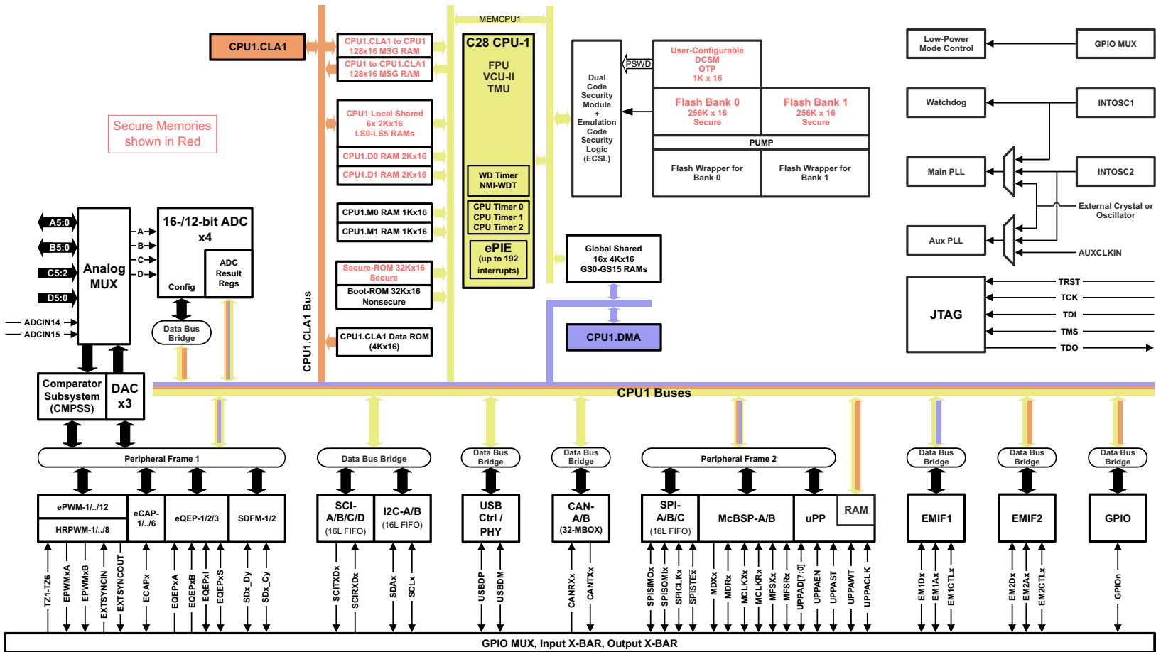
图 8-1. 功能方框图
