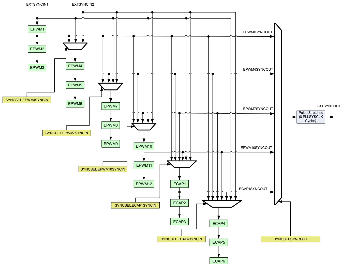
图 7-51. 同步链架构
