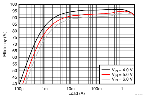
效率与输出电流间的关系；V OUT = 3.3V；PWM 和 PFM；f sw = 2.25MHz
