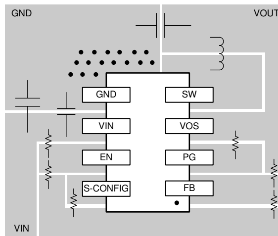
图 11-1. TPS629211-Q1 Layout
