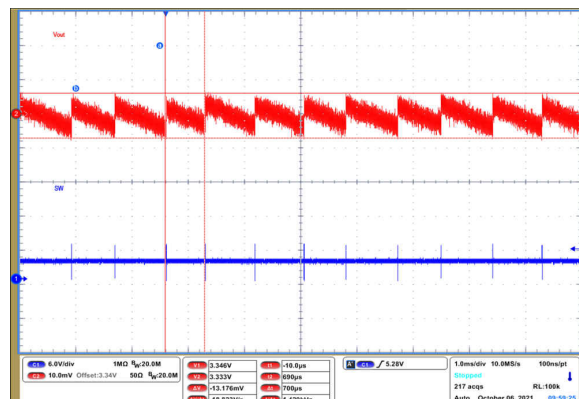
图 9-69. Output Voltage Ripple
