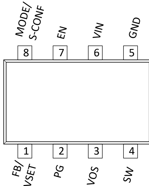
图 6-1. TPS629211-Q1 8-Pin DRL SOT-5X3 Pinout
