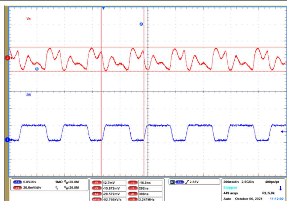
图 9-74. Input Voltage Ripple
