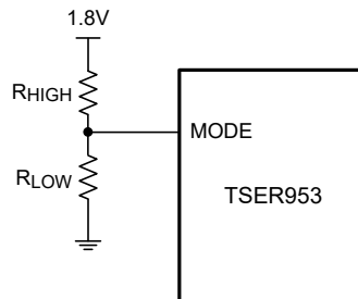
图 7-7. MODE Configuration
