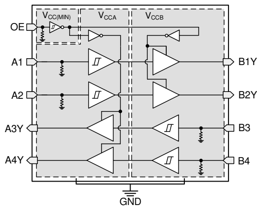
图 5-2. TXU0204 Functional Block Diagram
