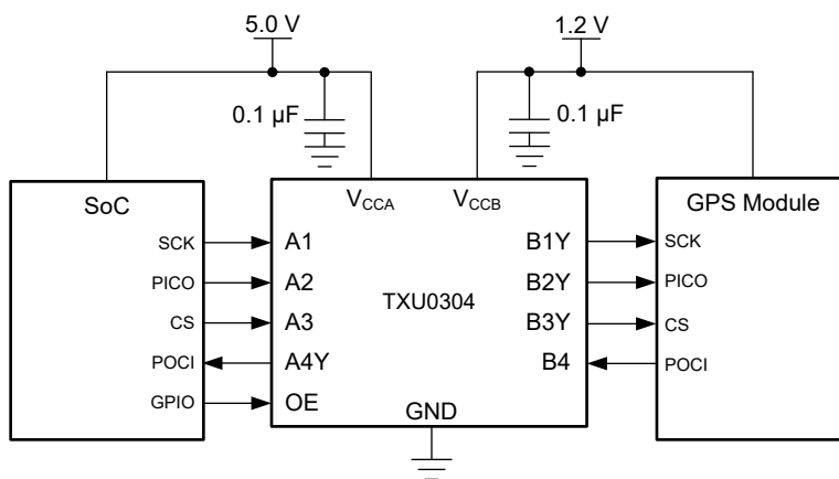
图 10-1. TXU0304 SPI Interface Application
