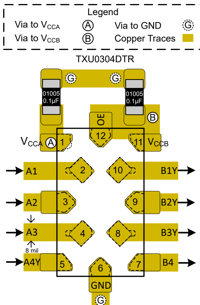
图 12-1. Layout Example - TXU0304
