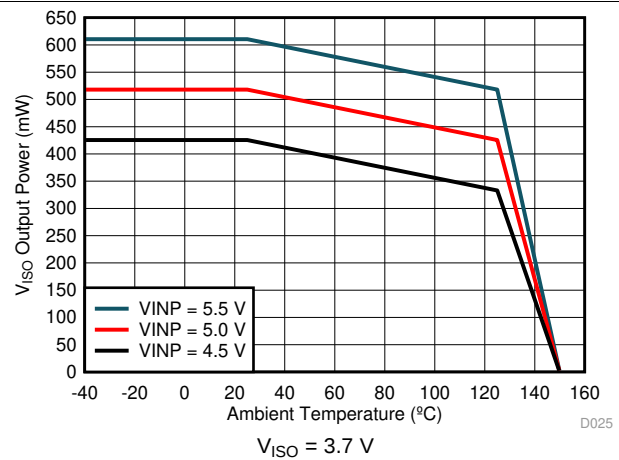
图 7. Maximum V_{ISO} Output Power vs. Temperature
