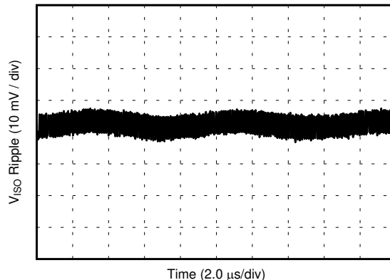
图 36. V_{ISO} Ripple, 3.3-V Output, 90% Load
