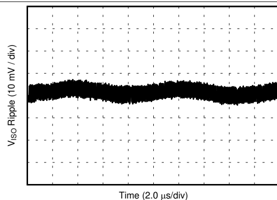
图 32. V ISO Ripple, 5.0-V Output, 90% Load
