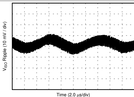
图 31. V ISO Ripple, 5.0-V Output, 10% Load
