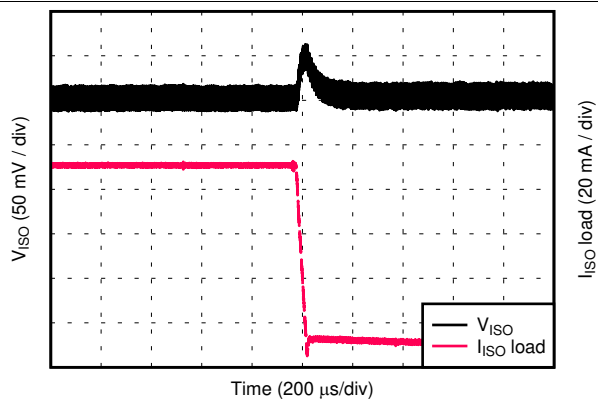
图 40. V_{ISO} Load Transient Response, 90% to 10% Load Step, 5.0-V Input, 5.0-V Output D044
