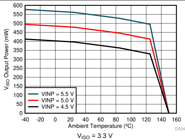
图 6. Maximum V_{ISO} Output Power vs. Temperature
