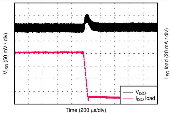
图 38. V_{ISO} Load Transient Response, 90% to 10% Load Step, 5.0-V Input, 5.4-V Output D042
