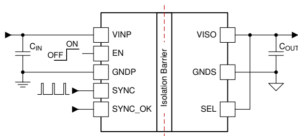
简化应用
