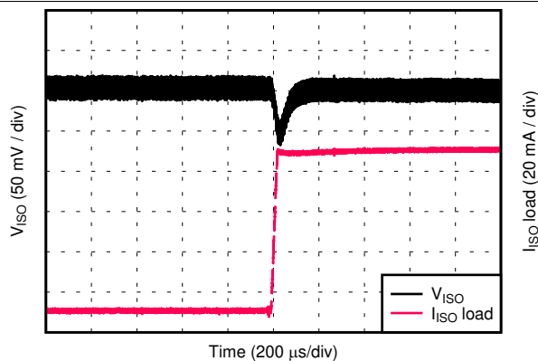
图 39. V_{ISO} Load Transient Response, 10% to 90% Load Step, 5.0-V Input, 5.0-V Output D043
