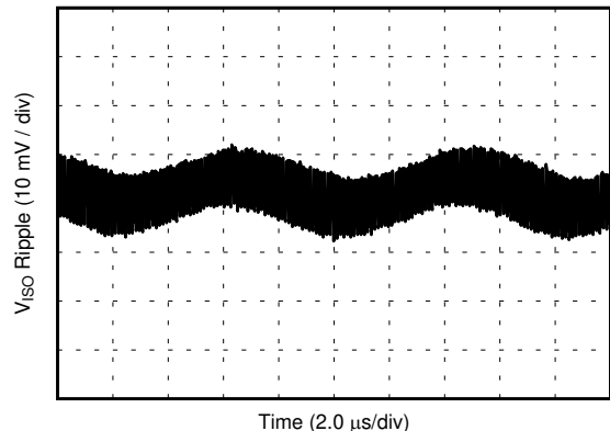
图 35. V_{ISO} Ripple, 3.3-V Output, 10% Load
