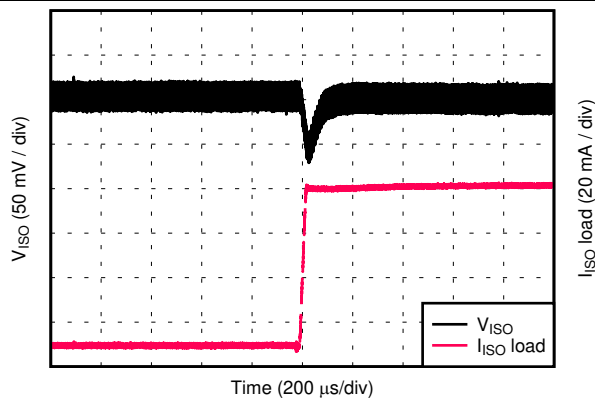
图 37. V_{ISO} Load Transient Response, 10% to 90% Load Step, 5.0-V Input, 5.4-V Output D041
