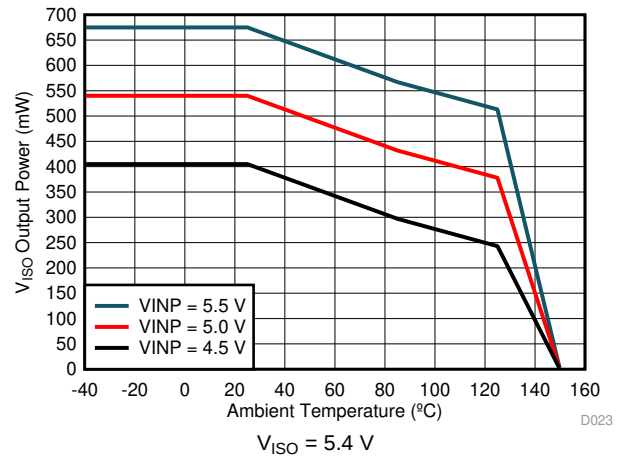
图 5. Maximum V_{ISO} Output Power vs. Temperature
