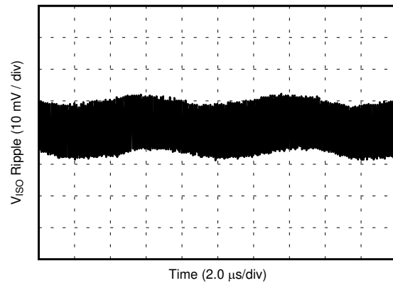
图 30. V ISO Ripple, 5.4-V Output, 90% Load
