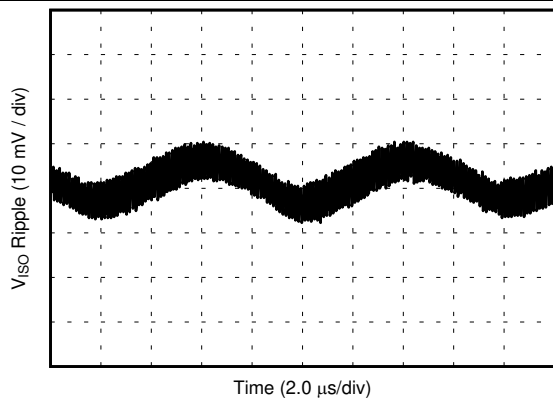
图 29. V ISO Ripple, 5.4-V Output, 10% Load
