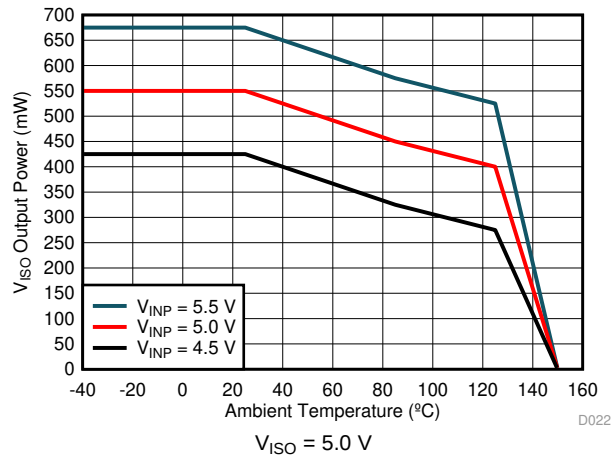
图 4. Maximum V_{ISO} Output Power vs. Temperature
