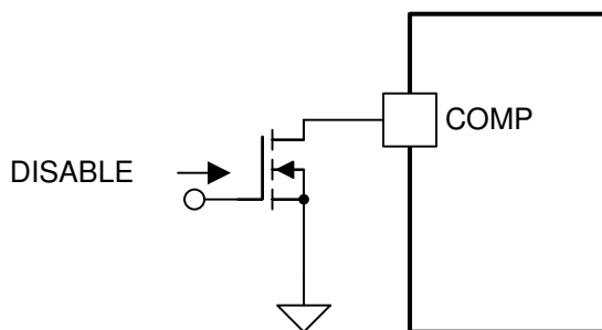
图 8-7. Disable Circuit
