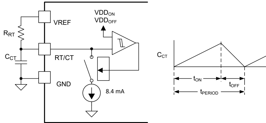
图 8-4. Oscillator Circuit
