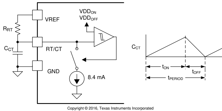
图 8-4. Oscillator Circuit
