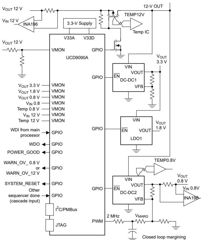
典型应用
